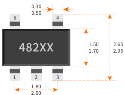
SOT-23-5L SO封装
