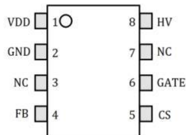
SOP-8俯视图
