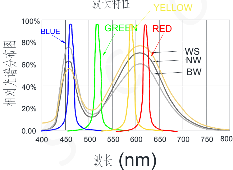
波长特性
