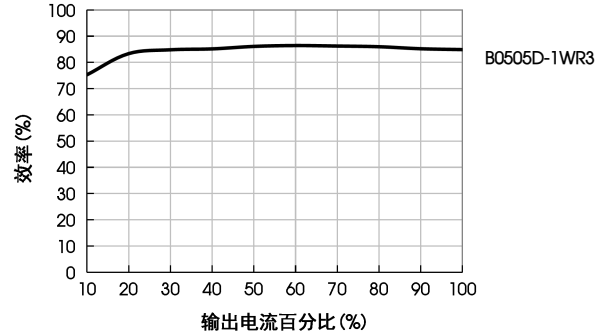
效率Vs输出负载 (Vin=5V)
