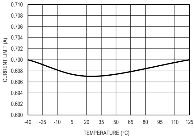
图 14. 输出限值值和温度的关系
