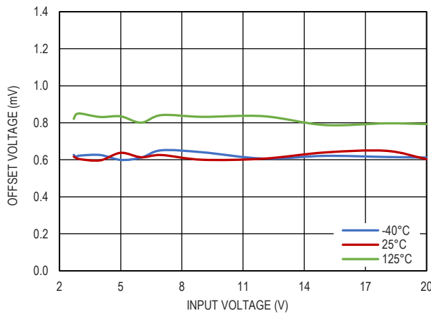
图 6. |V_{OUT}-V_{SET}| 和输入电压的关系, V_{OUT}=1.8V
