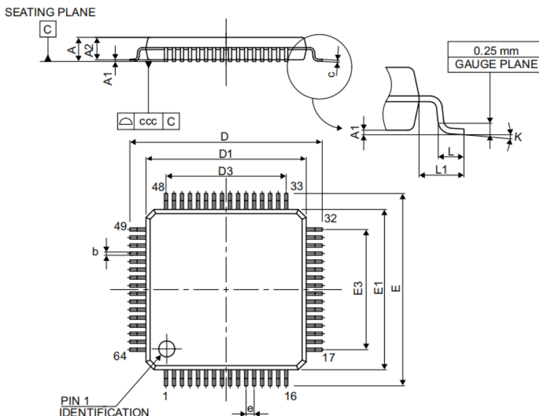
图 54 LQFP64，64 脚低剖面方形扁平封装图
