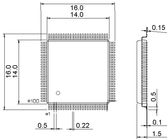
图 5-5 LQFP100 封装
