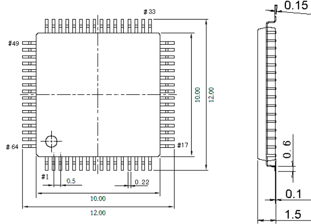
图 5-4 LQFP64M 封装
