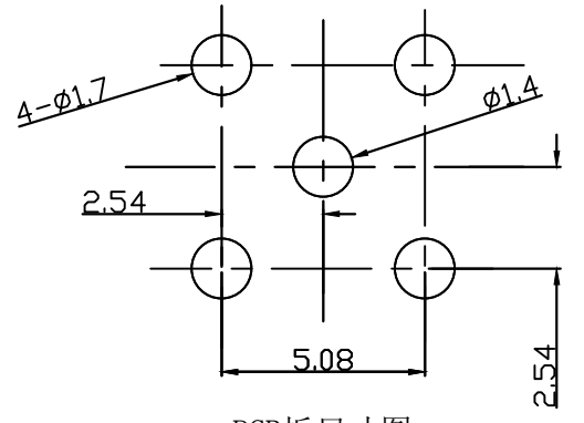
PCB板尺寸图
