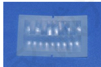
型号: 7805-1 尺寸: 56.7 * 35.8 焦距: 22mm 感应角度: 100^\circ 感应距离: 10m
