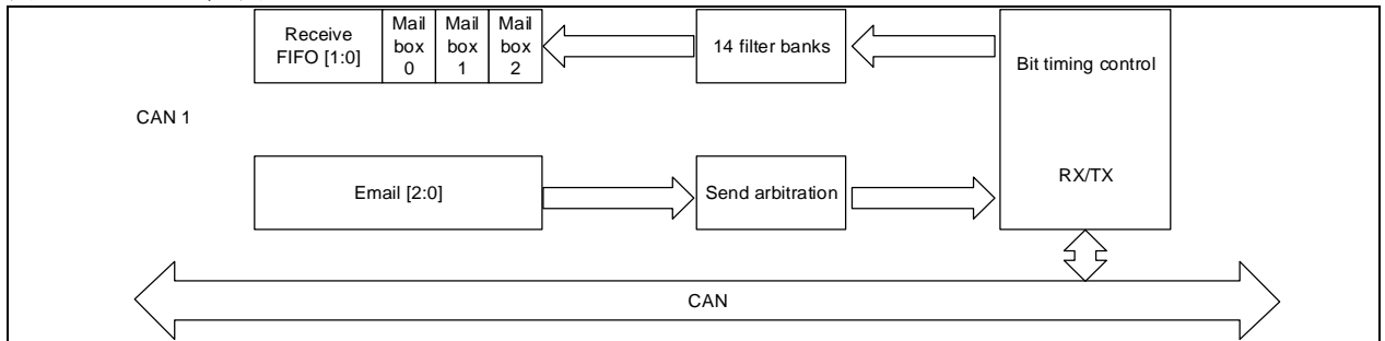
图 19-7 CAN 框图
