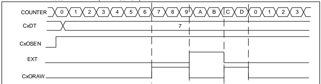
图 14-79 EXT清除 CxORAW(PWM模式 A)
