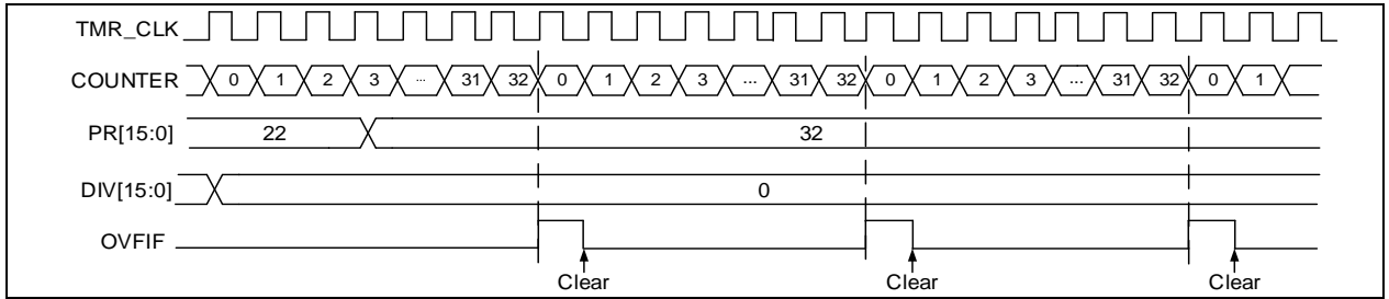
图 14-11 PRBEN=1时的溢出事件
