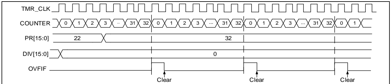
图 14-63 PRBEN=1时的溢出事件
