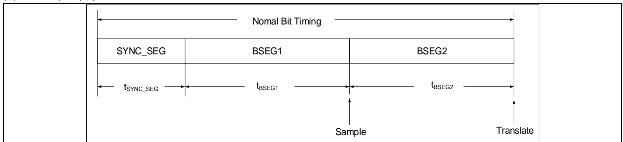
图 19-1 位时序
