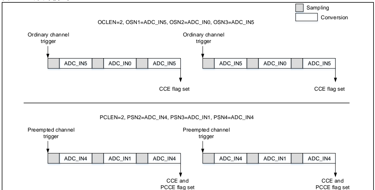
图 18-4 序列模式
