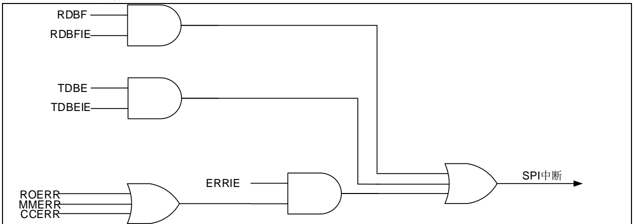
图 13-12 SPI中断
