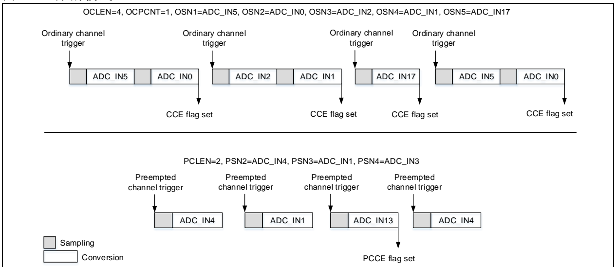
图 18-7 分割模式
