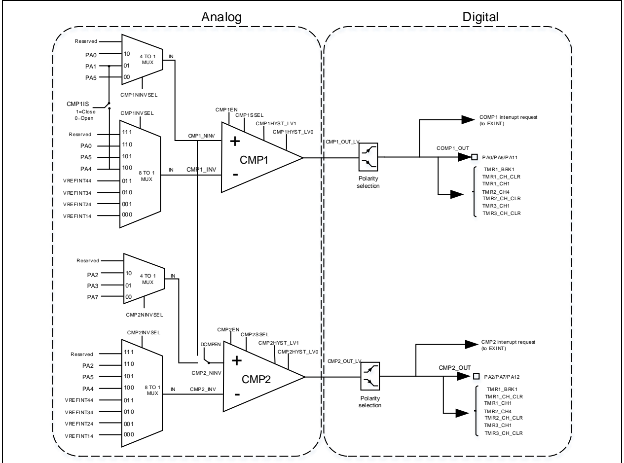
图 21-1 比较器的框图
