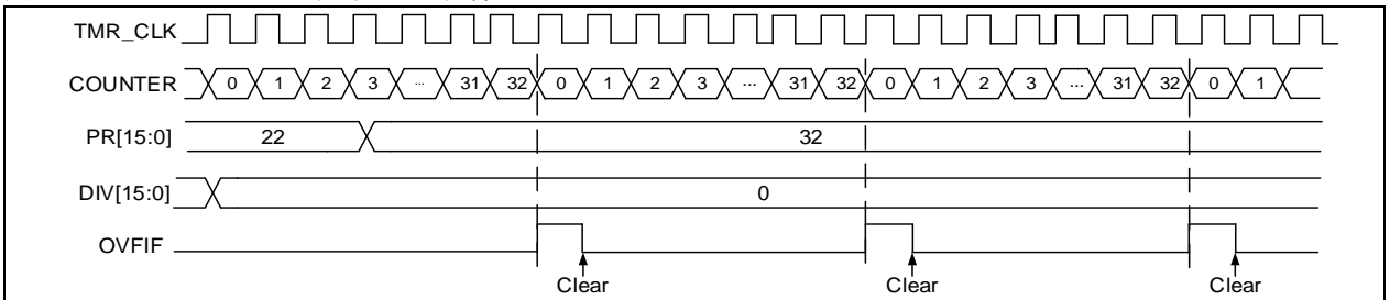
图 14-41 PRBEN=1时的溢出事件
