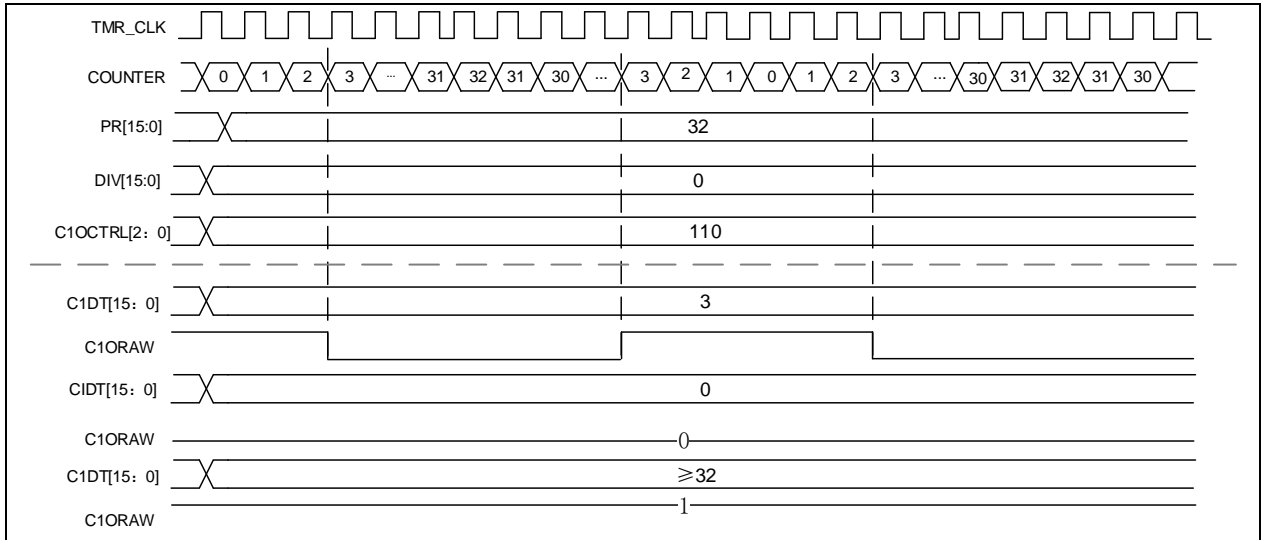
图 14-24 单周期模式
