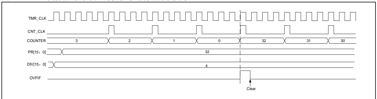
图 14-12 计数器时序图, 内部时钟分频因子为 4
