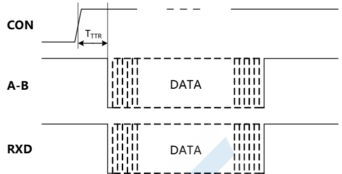
图 2. TD(3)511D485H模块数据接收时序图
