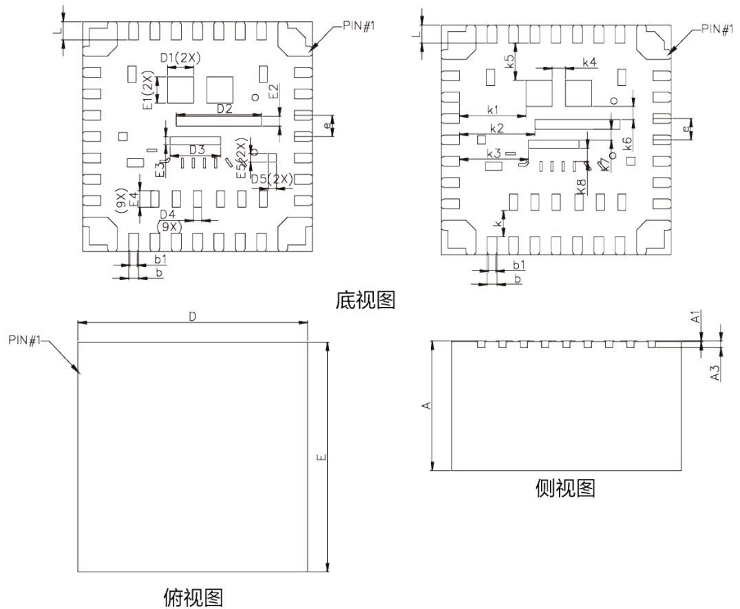
图 6-2 结构尺寸图
