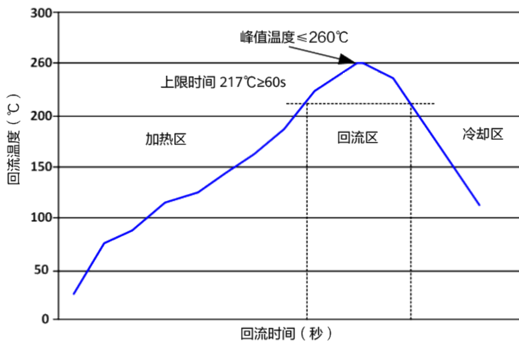
图 10-2 推荐无铅焊接回流曲线
