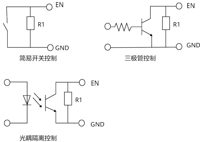
图 6-4 EN 引脚控制方式推荐图
