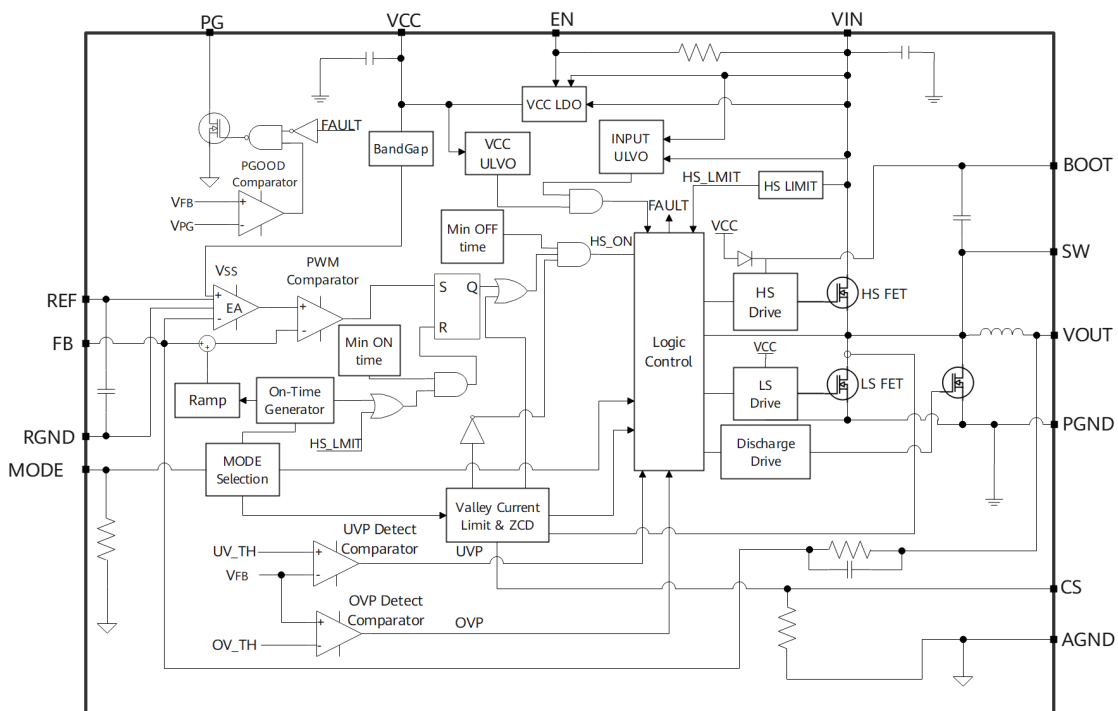
图 3-1 原理框图
