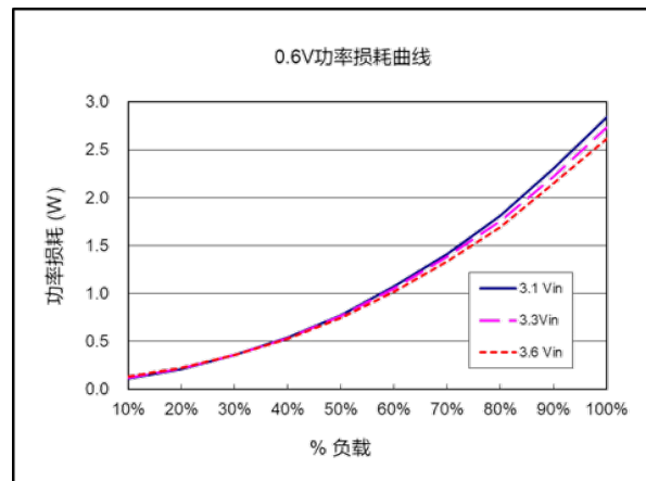
功率损耗曲线 ( V_{nom}=3.3V, V_{out}=0.6V )
