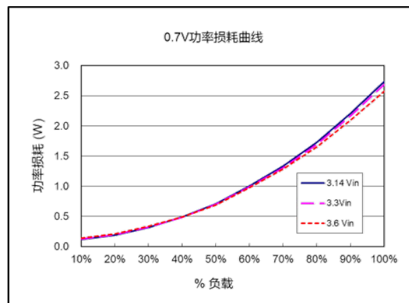
功率损耗曲线 ( V_{nom}=3.3V, V_{out}=0.7V )
