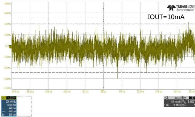
图 13. 10Hz-100kHz 噪声
