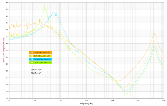
图 12. 纹波抑制比与频率
