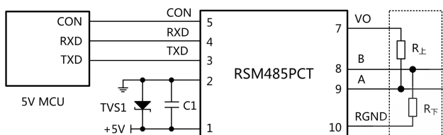
图 3. MCU 5V 供电应用电路
