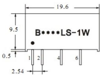
正视图
