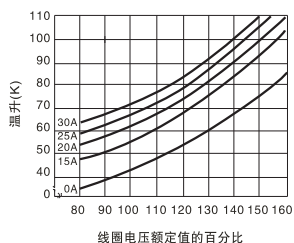
线圈温升
