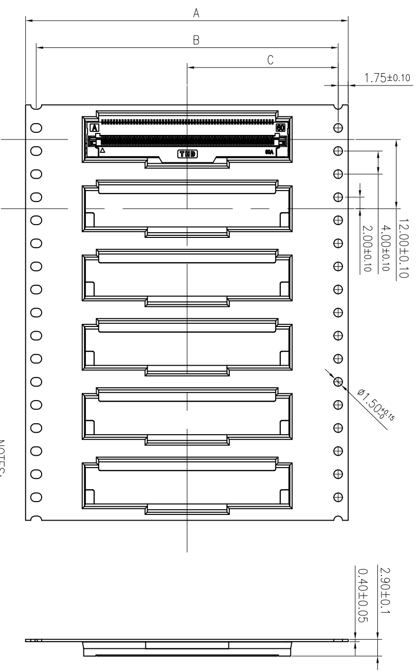
REEL DIM
