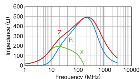
MMZ1608S202ATD25
