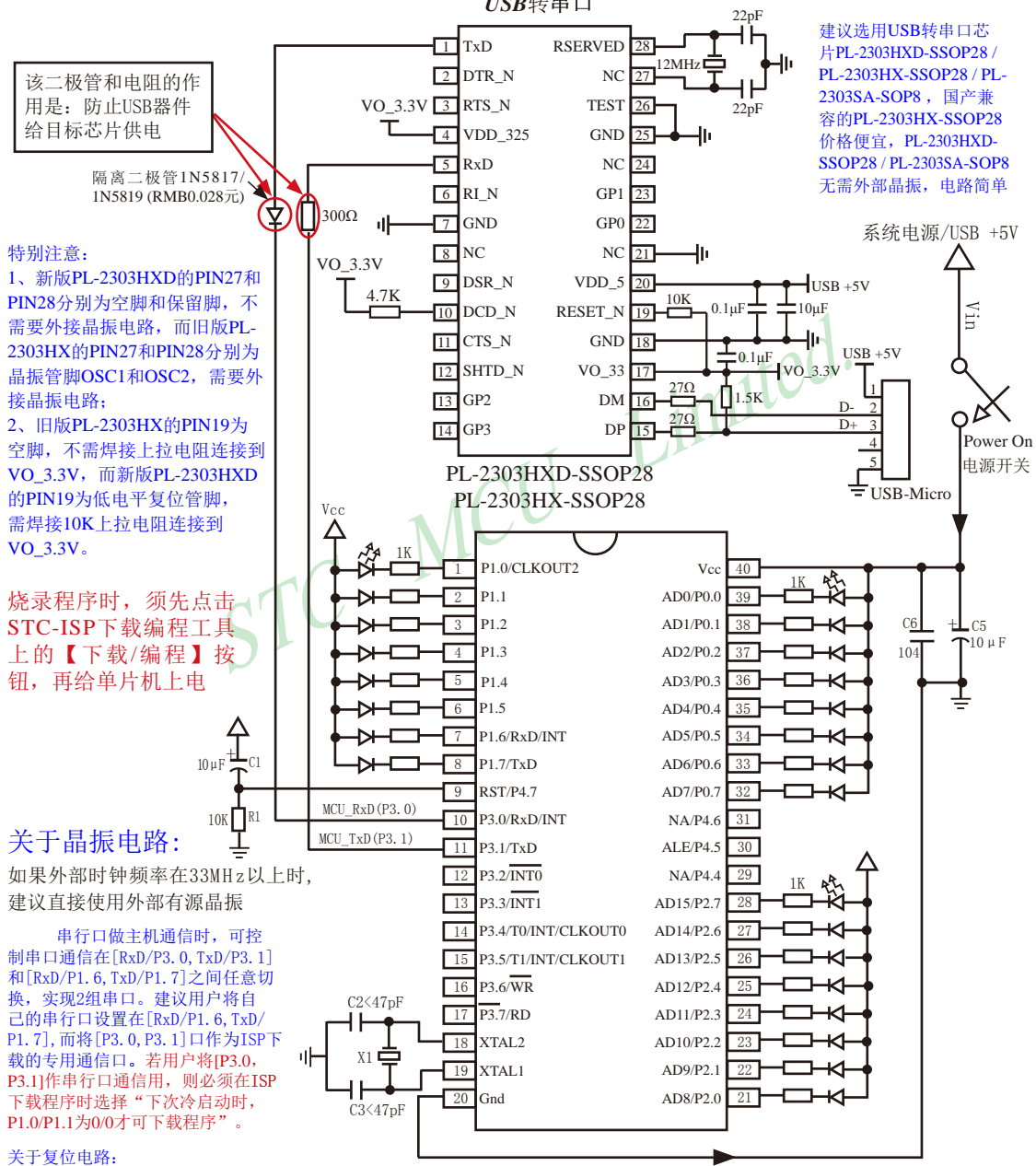
应用线路图
