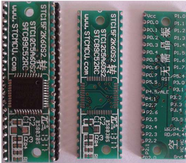
完整转换板
