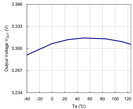
VR=3.3V
