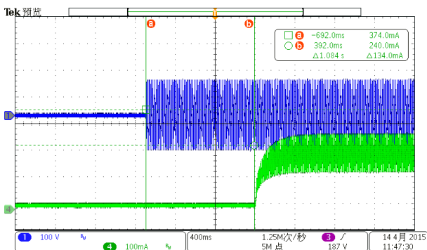
90Vac CH3:Vin-ac CH4: Io
