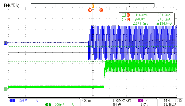
264Vac CH1:Vin CH4: Io
