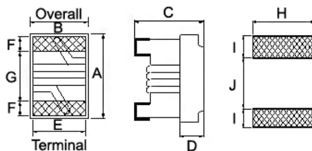
CM0603
