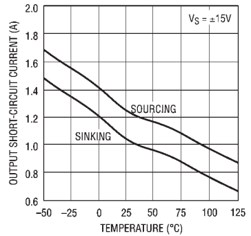
输出短路电流与结温的关系曲线
