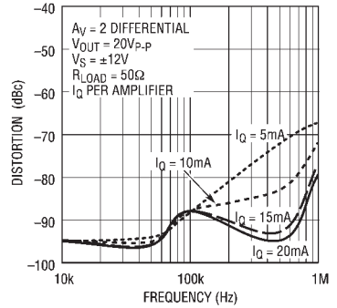
二次谐波失真与频率的关系曲线
