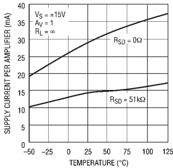
电源电流与环境温度的关系曲线
