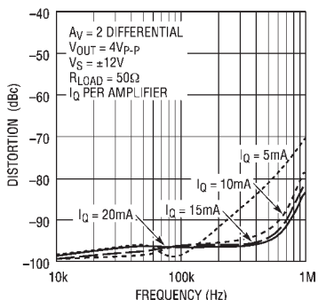
二次谐波失真与频率的关系曲线
