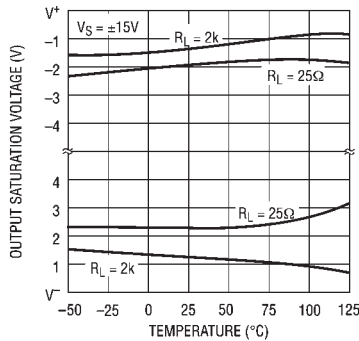
输出饱和电压与结温的关系曲线
