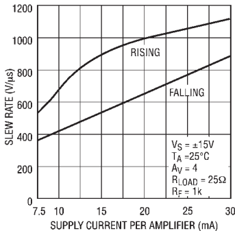
转换速率与电源电流的关系曲线
