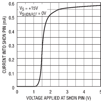
SHDN引脚电流与电压的关系曲线
