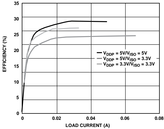
图4. 5 V/5 V、5 V/3.3 V和3.3 V/3.3 V的典型电源效率
