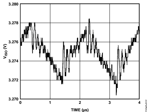
图12. V_{ISO} = 3.3V 输出电压典型纹波, 90%负载
