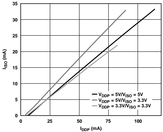
图6. 5 V/5 V、5 V/3.3 V和3.3 V/3.3 V时典型隔离输出电源电流 I_{ISO} 与外部负载的关系
