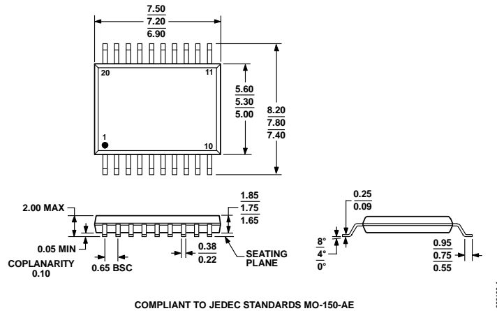
图22. 20引脚紧缩小型封装[SSOP] (RS-20)
