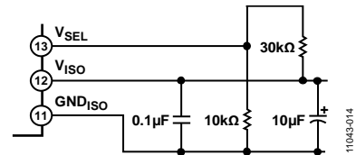
图17. V_{ISO} 偏置和旁路组件
