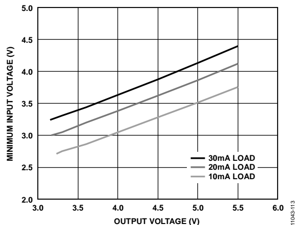
图13. 输出电压和所需输入电压之间的关系, 负载未滿, 保持PWM中占空系数大于80%
