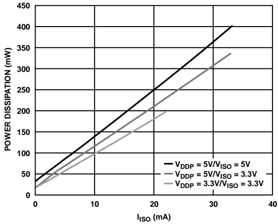
图5. 典型总功耗与 I_{ISO} 的关系
