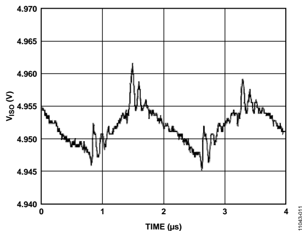
图11. V_{ISO} = 5V 输出电压典型纹波, 90%负载
