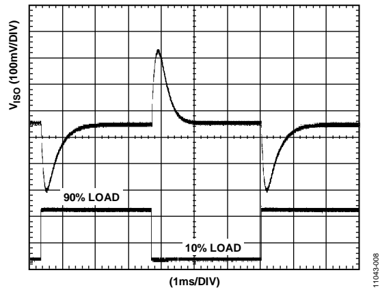
图8. 典型 V_{ISO} 瞬态负载响应，5 V输入，5 V输出，10%至90%负载阶跃
