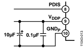
图16. V_{DDP} 偏置和旁路组件
