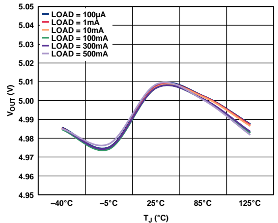
图15. 输出电压与结温的关系 (VOUT = 5 V)
