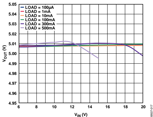
图17. 输出电压与输入电压的关系( V_{OUT} = 5\text{ V} )
