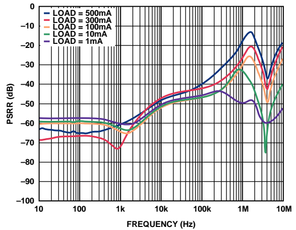
图39. 电源抑制比与频率的关系( V_{OUT} = 5\text{ V} , V_{IN} = 5.5\text{ V} )
