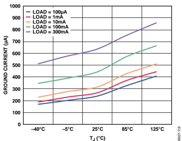
图18. 接地电流与结温的关系( V_{OUT} = 5\text{ V} )
