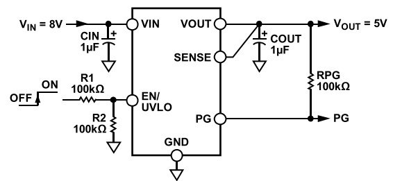
图1. 提供5 V固定输出电压的ADP7104
