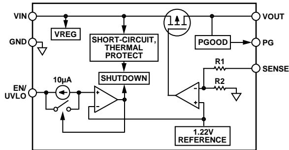
图59. 固定输出电压型号内部框图
