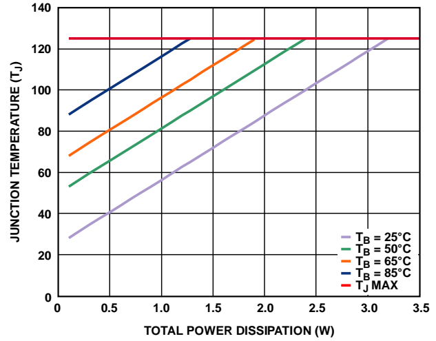
图77. SOIC封装
