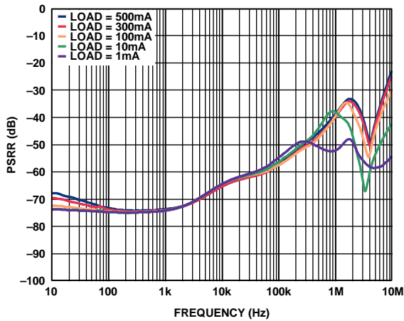
图37. 电源抑制比与频率的关系( V_{OUT} = 5\text{ V} , V_{IN} = 6.5\text{ V} )
