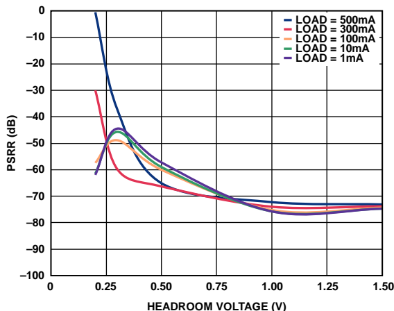
图44. 电源抑制比与裕量电压的关系(100 Hz, V_{OUT} = 5V )
