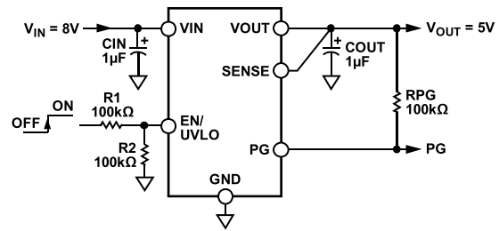
图65 EN引脚的典型分压器
