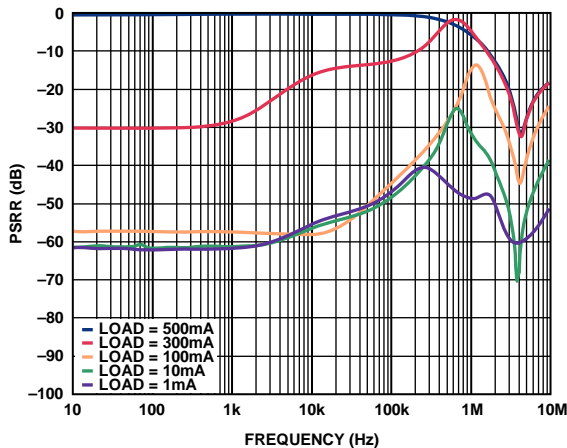
图41. 电源抑制比与频率的关系( V_{OUT} = 5V , V_{IN} = 5.2V )
