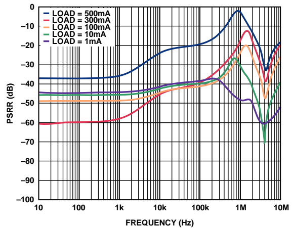
图40. 电源抑制比与频率的关系( V_{OUT} = 5\text{ V} , V_{IN} = 5.3\text{ V} )
