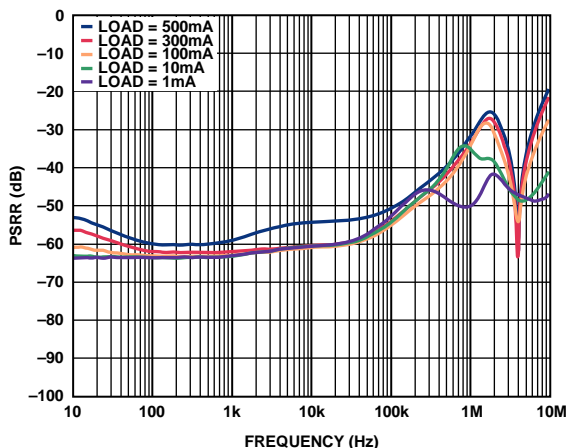
图42. 电源抑制比与频率的关系( V_{OUT} = 5V , V_{IN} = 6V , 可调)
