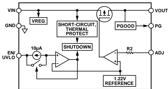
图60. 可选输出电压型号内部框图
