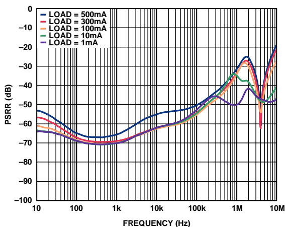
图43. 电源抑制比与频率的关系( V_{OUT} = 5V , V_{IN} = 6V , 可调并带降噪电路)
