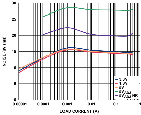
图48. 输出噪声与负载电流和输出电压的关系( C_{OUT} = 1 \mu F )
