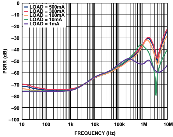
图35. 电源抑制比与频率的关系( V_{OUT} = 3.3\text{ V} , V_{IN} = 4.3\text{ V} )
