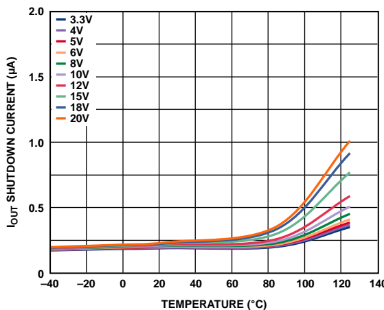
图32. 反相输入电流与温度的关系( V_{IN} = 0\text{ V} , V_{OUT} 为差分电压)
