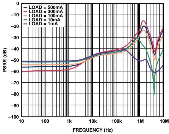
图36. 电源抑制比与频率的关系( V_{OUT} = 3.3\text{ V} , V_{IN} = 3.8\text{ V} )
