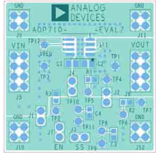
图79. SOIC PCB布局示例
