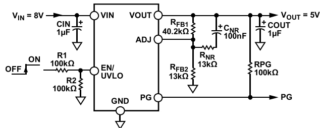
图69. 更改可调输出LDO以降低噪声
