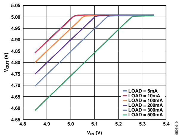
图21. 低压差下输出电压与输入电压的关系
