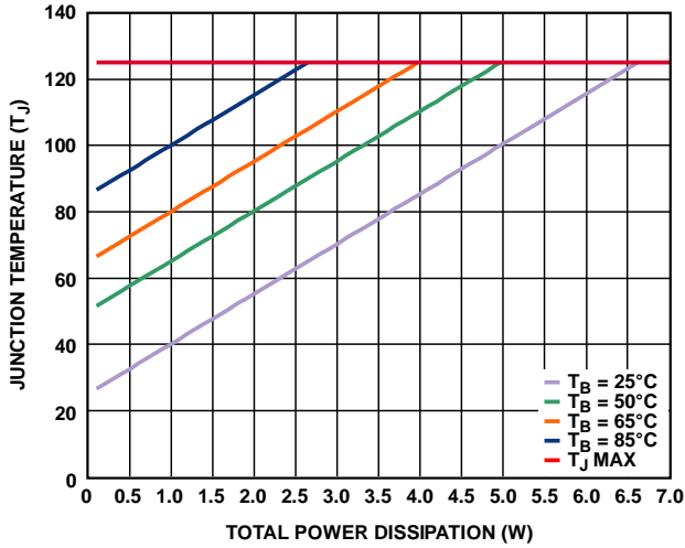
图76. LFCSP封装
