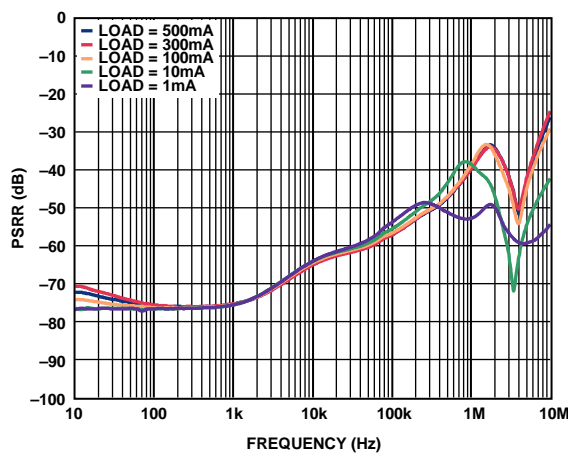
图33. 电源抑制比与频率的关系( V_{OUT} = 1.8\text{ V} , V_{IN} = 3.3\text{ V} )
