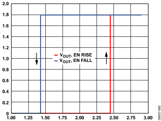
图64. 对EN引脚工作方式的典型VOUT响应
