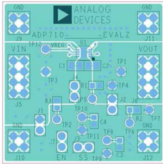
图78. LFCSP PCB布局示例
