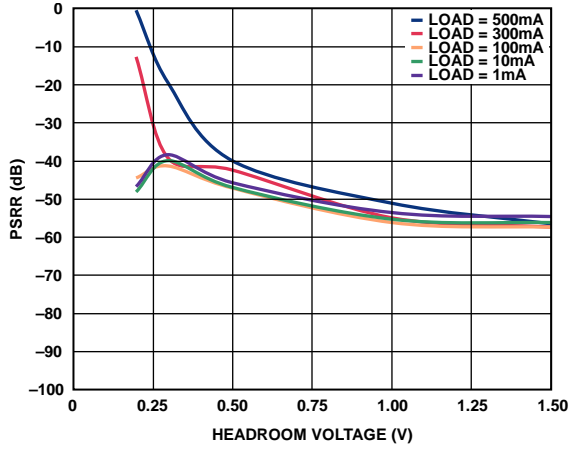
图47. 电源抑制比与裕量电压的关系(100 kHz, V_{OUT} = 5 V )
