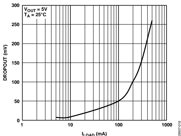
图20. 压差与负载电流的关系( V_{OUT} = 5\text{ V} )
