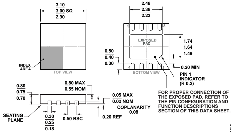
图80. 8引脚引脚架构芯片级封装[LFCSP_WD] 3 mm x 3 mm, 超薄体, 双排引脚 (CP-8-5)
