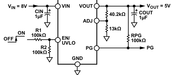
图2. 提供5 V可调输出电压的ADP7104
