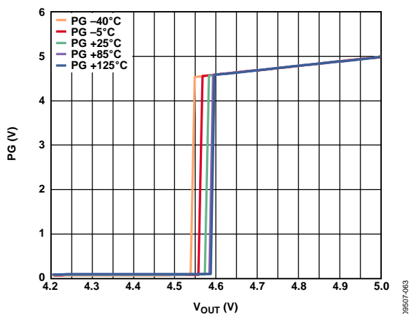
图68. 典型电源良好阈值与温度的关系( V_{OUT} 下降)
