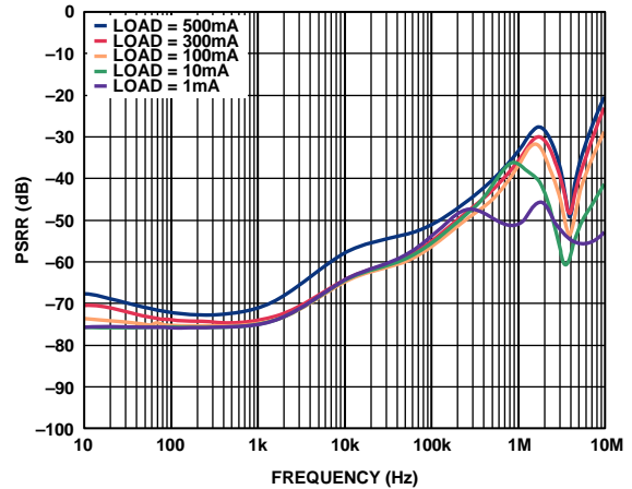
图38. 电源抑制比与频率的关系( V_{OUT} = 5\text{ V} , V_{IN} = 6\text{ V} )
