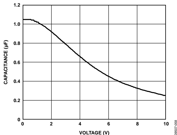
图63. 电容与电压关系特性
