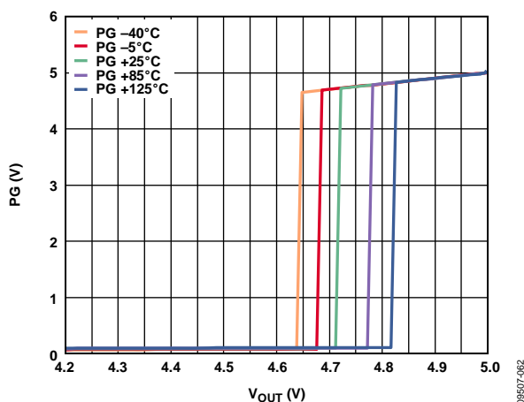
图67. 典型电源良好阈值与温度的关系( V_{OUT} 上升)
