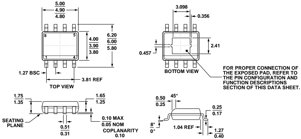
图81. 8引脚标准小型封装, 带裸露焊盘[SOIC_N_EP] 窄体 (RD-8-2)
