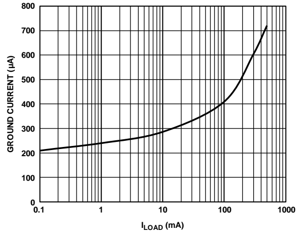
图9. 接地电流与负载电流的关系
