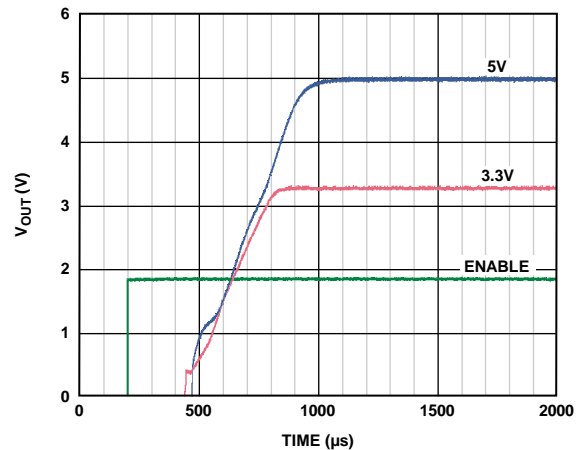
图66. 典型启动性能
