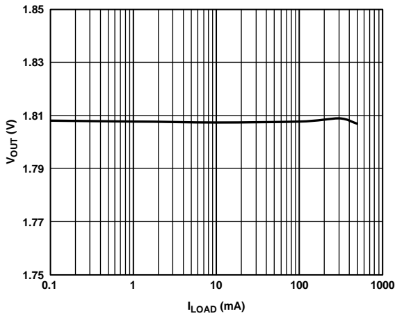
图24. 输出电压与负载电流的关系( V_{OUT} = 1.8\text{ V} )
