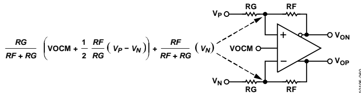
图53. AD8476内部运放输入端电压
