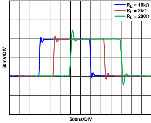
图29. 不同阻性负载下的小信号阶跃响应( V_s = \pm 5V )
