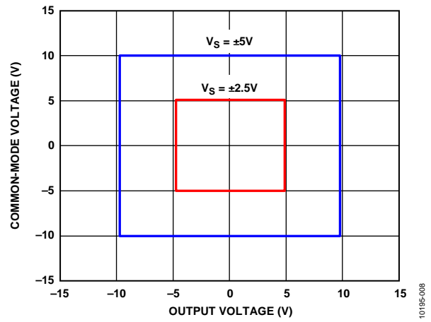
图8. 输入共模电压与输出电压的关系 ( V_S = 5V 和 \pm 2.5V )
