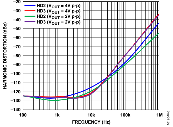
图39. 不同 V_{OUT,dm} 下谐波失真与频率的关系
