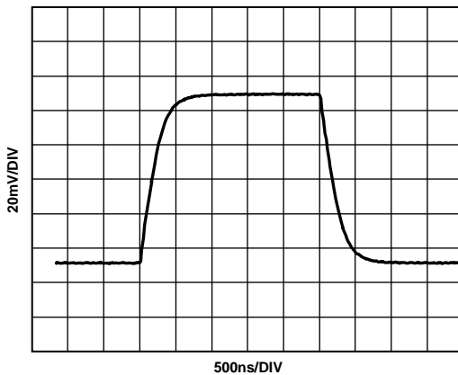
图30. 不同容性负载下的小信号阶跃响应( V_s = \pm 5V )
