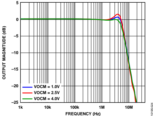
图23. 不同V OCM 电平下的小信号频率响应
