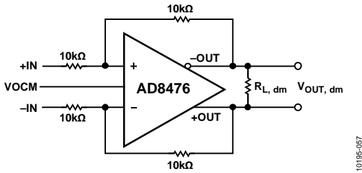
图50. 信号和电路定义
