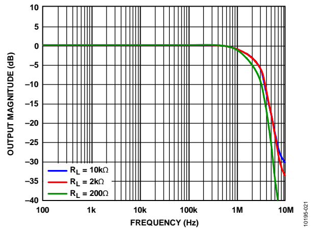
图21. 不同负载下的大信号频率响应
