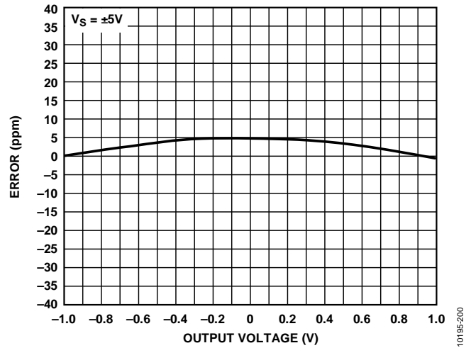
图44. 增益非线性度
