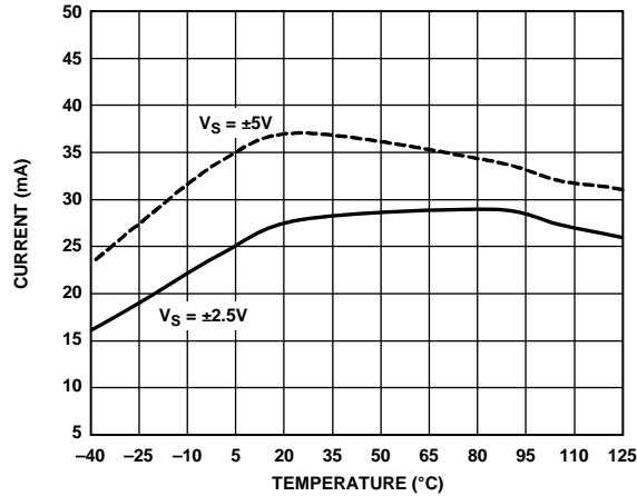
图14. 短路电流与温度的关系
