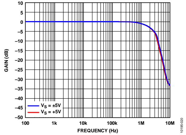
图20. 不同电源下的大信号频率响应
