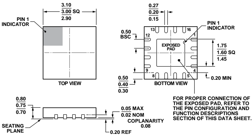
图58. 16引脚引线框芯片级封装[LFCSP_WQ] 3 mm x 3 mm, 超薄体 (CP-16-25)
