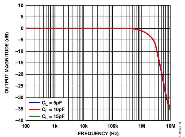
图22. 不同容性负载下的大信号频率响应
