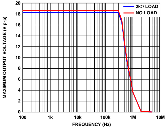
图11. 最大输出电压与频率的关系
