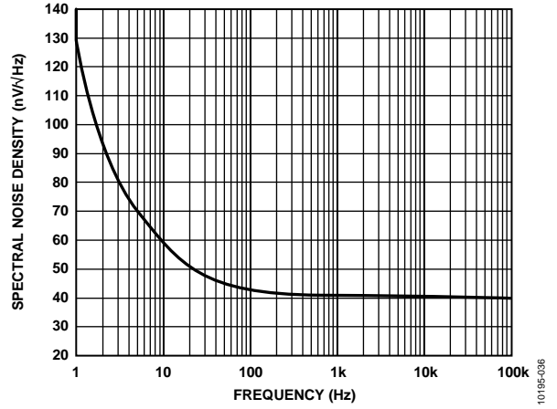
图38. 电压噪声密度与频率的关系
