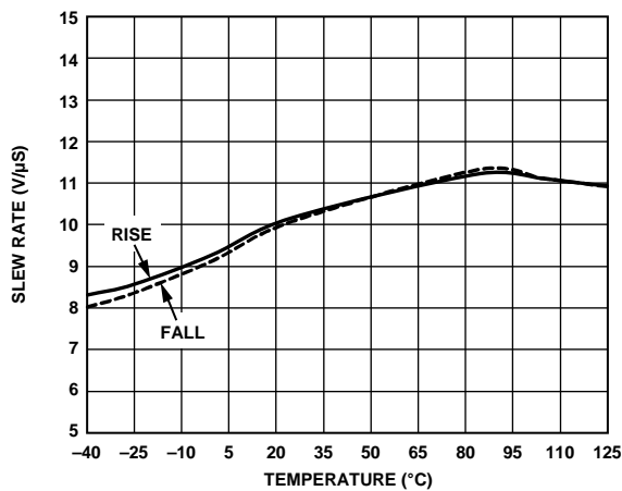
图13. 压摆率与温度的关系
