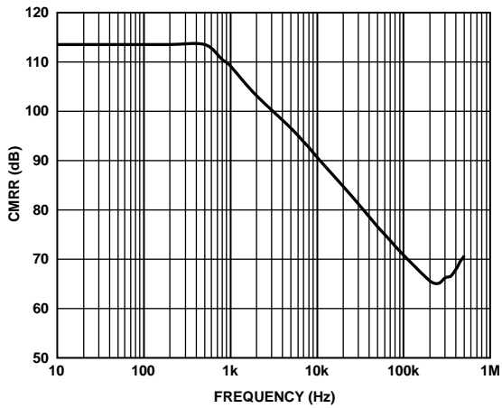
图4. 典型CMRR与频率的关系
