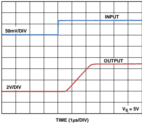
图15. 差分过载恢复时间(上升, V_S = 5V )
