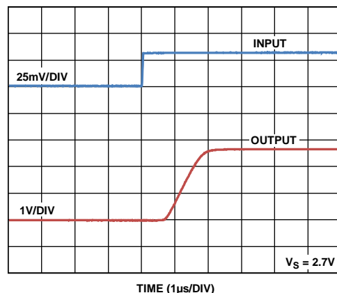
图14. 差分过载恢复时间(上升, V_S = 2.7V )
