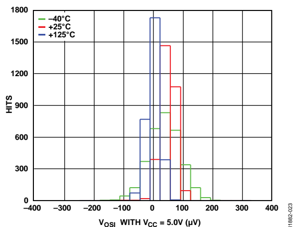
图23. 失调电压分布
