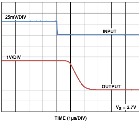
图16. 差分过载恢复时间(下降, V_S = 2.7V )
