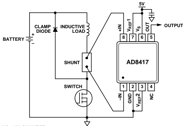
图34. 低边开关
