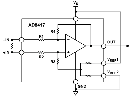
图30. 平分电源
