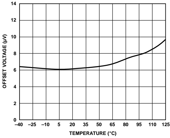
图3. 典型失调电压漂移与温度的关系
