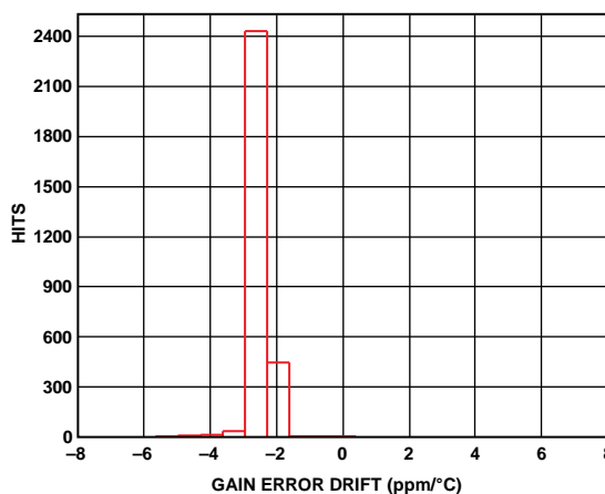
图25. 增益误差漂移分布图
