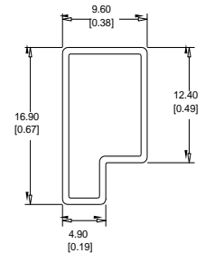
注: 单位 (Unit): mm[inch] 未注明公差: x.x±0.5mm[x.x±0.020inch] 0.x±0.2mm[0.x±0.008inch]
