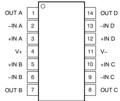
封装:HGV4333A 14 引脚 TSSOP 俯视图
