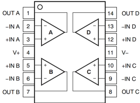
封装:HGV4333A 14 引脚 SOP 俯视图
