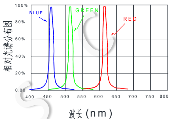
波长特性
