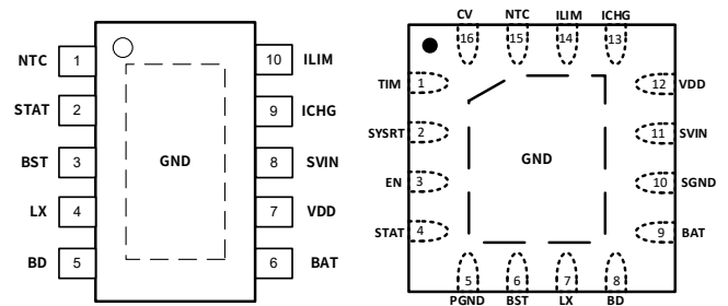
图3. 引脚排列
