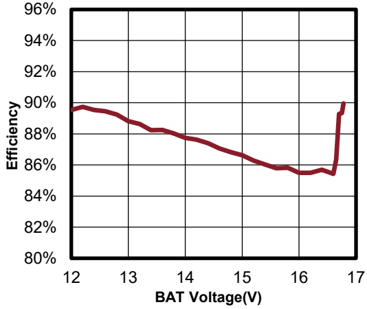
Figure 10.1.a R_{ICHG}=1.3K , 恒流和恒压充电阶段效率
