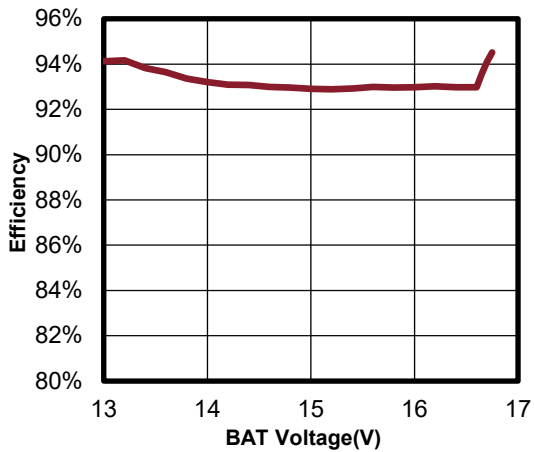
Figure 10.2.a R_{ICHG}=0.5K , 恒流和恒压充电阶段效率
