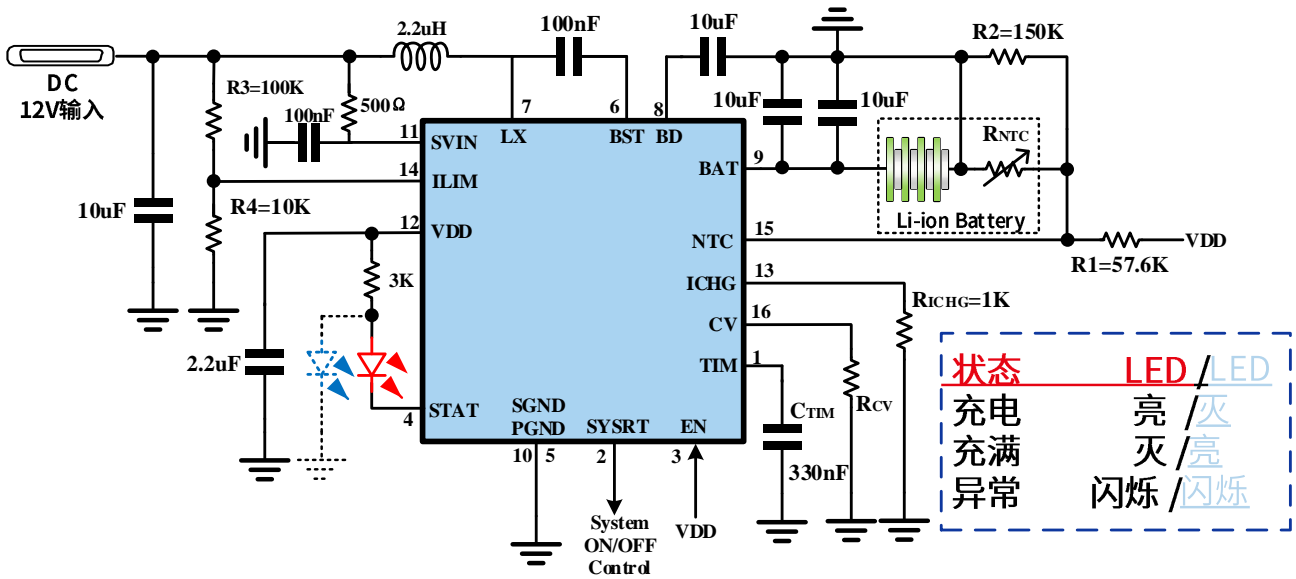
图 3. 55184 版本 DC 12V 适配器充电 (适应最低 11V DC 适配器; 电池充电温度为 0°C~60°C)
