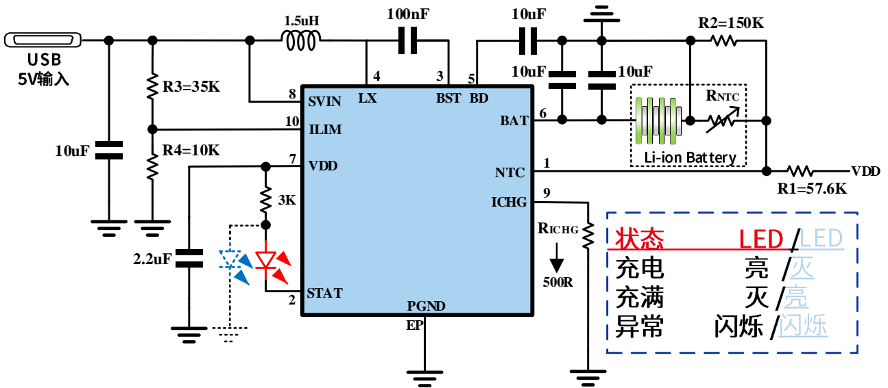
图 2.b. 55184 ESSOP10 版本 USB 5V 适配器充电 (适应最低 4.5V USB 适配器; 电池充电温度为 0°C~60°C)
