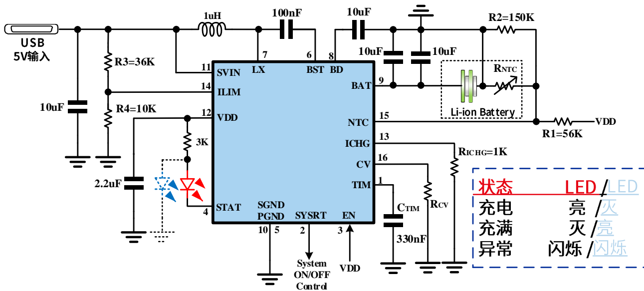
图 2.a. 55182 QFN 版本典型应用 1A 充电 (适应 4.5V USB; 电池充电温度为 0°C~60°C)
