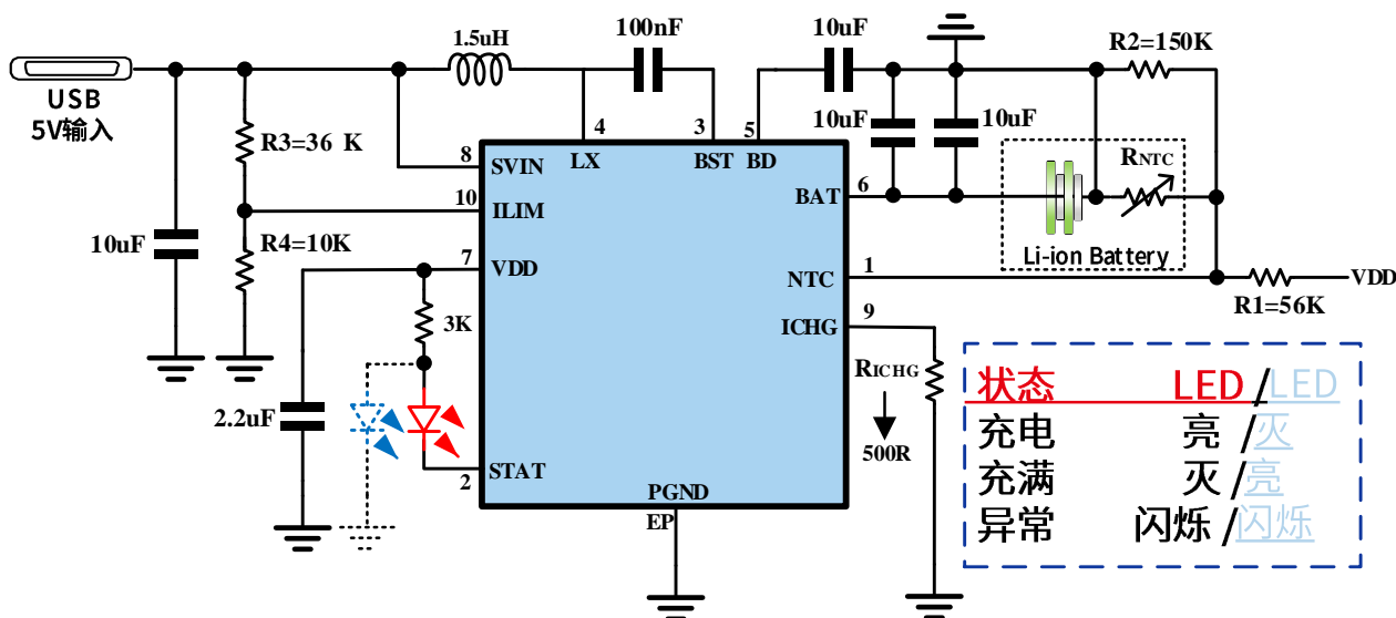
图 2.b. 55182 ESSOP10 版本 2A 充电 (适应 4.5V USB; 电池充电温度为 0°C~60°C)
