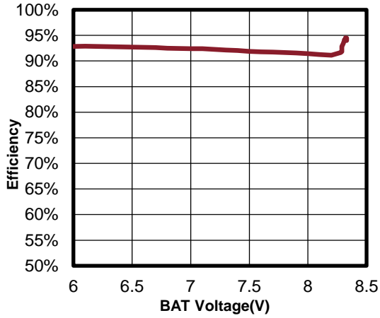
Figure 10.1.a R_{CHG}=1K , 恒流和恒压充电阶段效率
