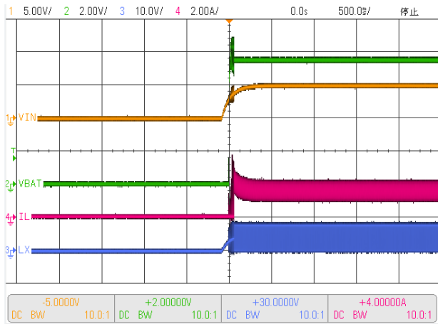
Figure 10.2.a 恒流充电 (CC) 上电波形
