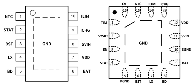
图 4. 引脚排列
