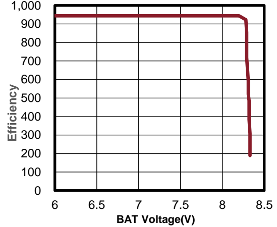
Figure 10.1.b R_{CHG}=1K , 恒流和恒压充电电流
