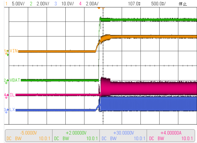
Figure 10.2.c 恒压充电 (CV) 上电波形
