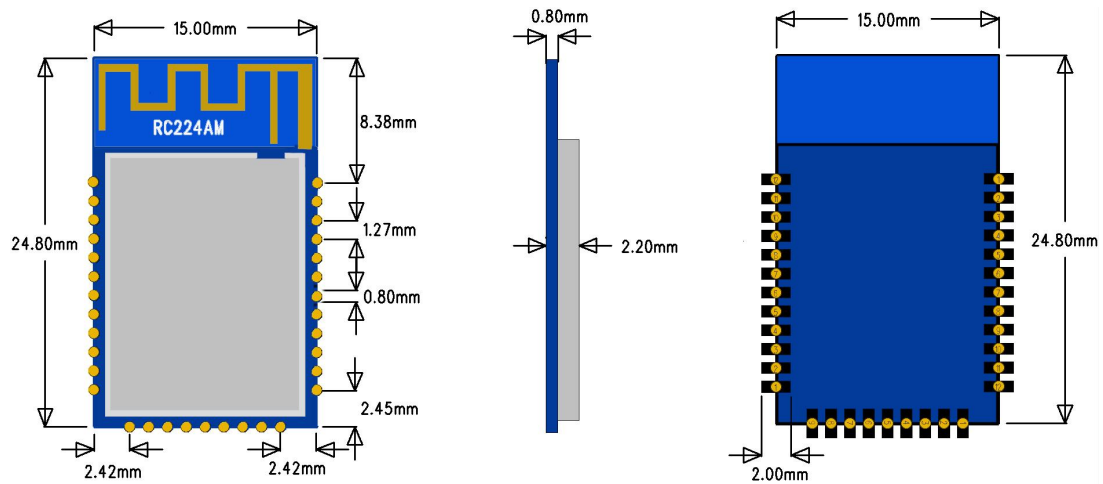
图 2. 模块尺寸图
