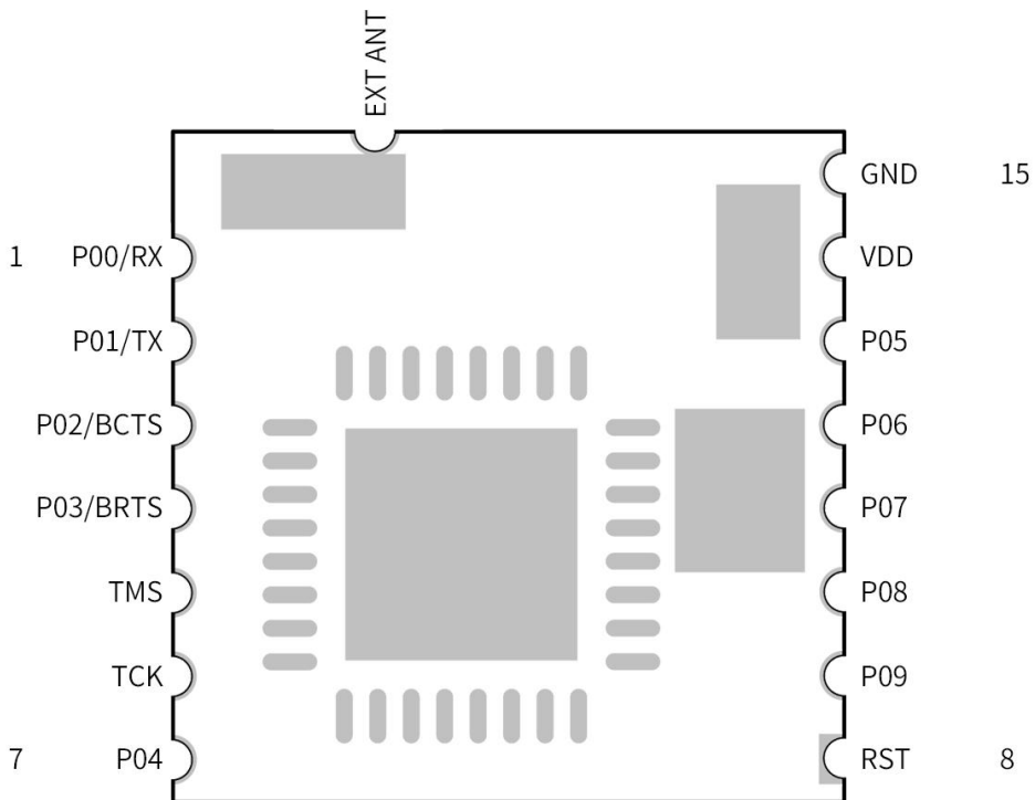
图6 模块引脚图
