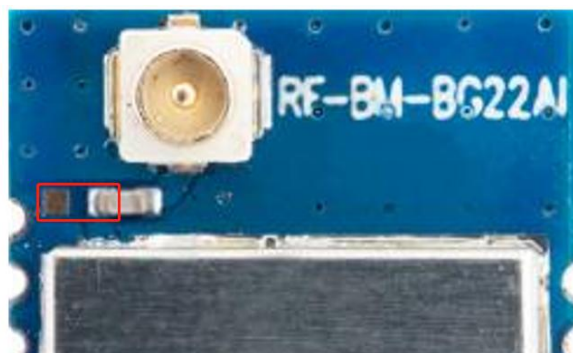
图 5. 天线输出方式更改
