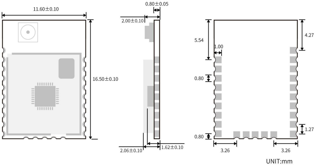
图 2. 尺寸图
