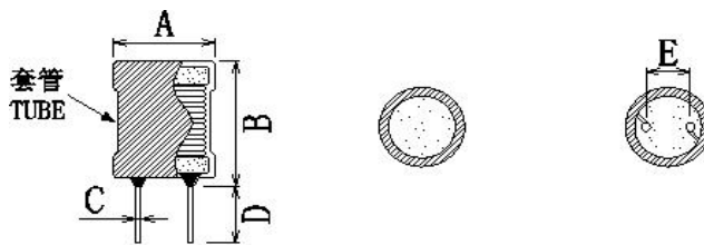
正视图 FRONT VIEW 顶视图 TOP VIEW 底视图 BOTTOM VIEW
