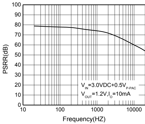
PSRR
