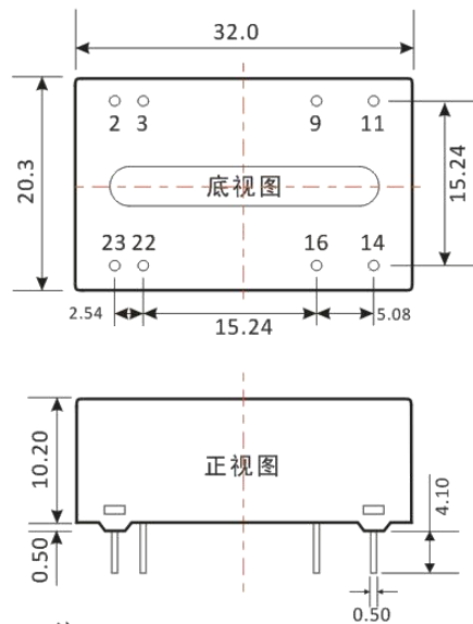
第一角投影示意图
