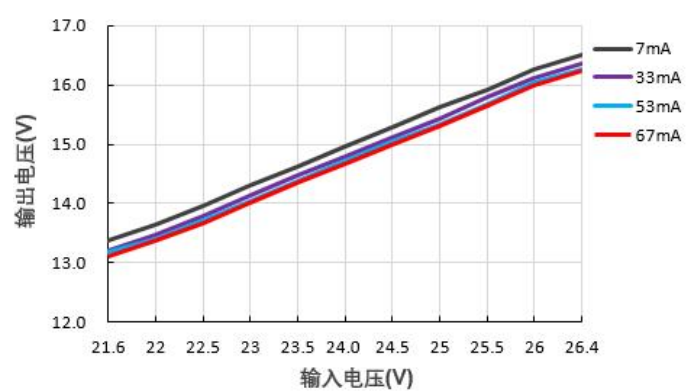
输出电压 VS 输入电压 (B2415S-1W)
