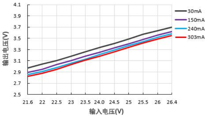
输出电压 VS 输入电压 (B2403S-1W)
