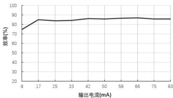
效率 VS 输出电流 (B0512S-1W@Vin=5V)
