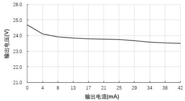
输出电压 VS 输出电流 (B1224S-1W@Vin=12V)
