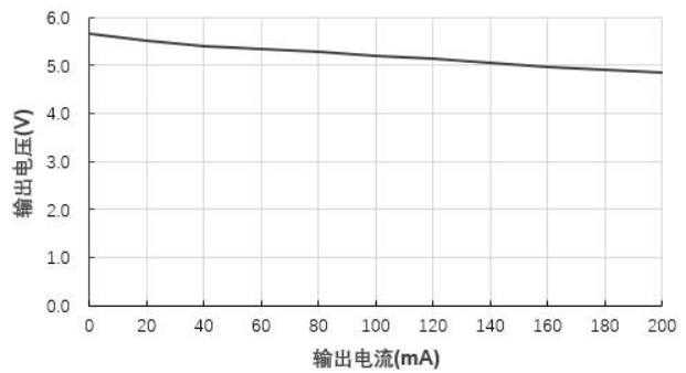
输出电压 VS 输出电流 (B0305S-1W@Vin=3.3V)
