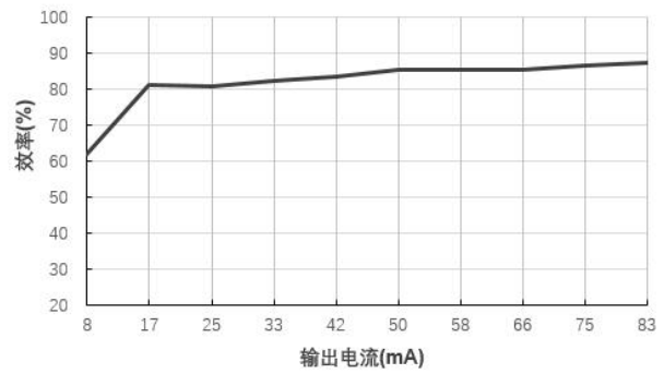
效率 VS 输出电流 (B1212S-1W@Vin=12V)
