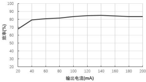
效率 VS 输出电流 (B1205S-1W@Vin=12V)
