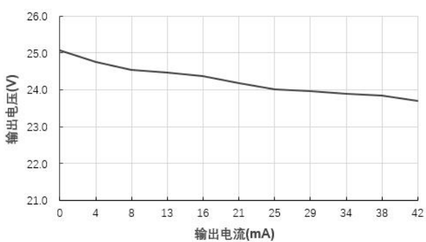
输出电压 VS 输出电流 (B0524S-1W@Vin=5V)
