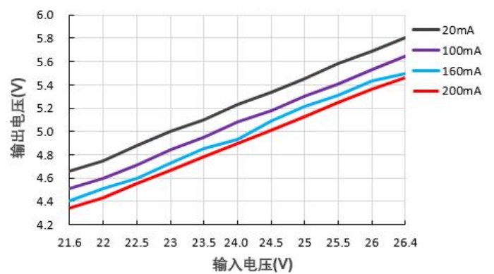
输出电压 VS 输入电压 (B2405S-1W)
