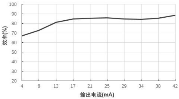
效率 VS 输出电流 (B2424S-1W@Vin=24V)
