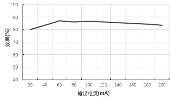
效率 VS 输出电流 (B0505S-1W@Vin=5V)
