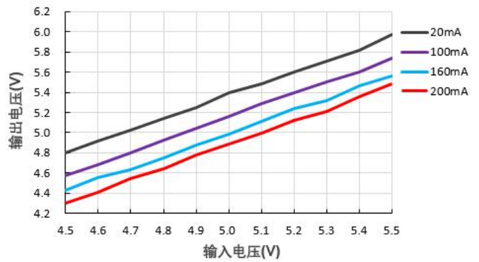
输出电压 VS 输入电压 (B0505S-1W)
