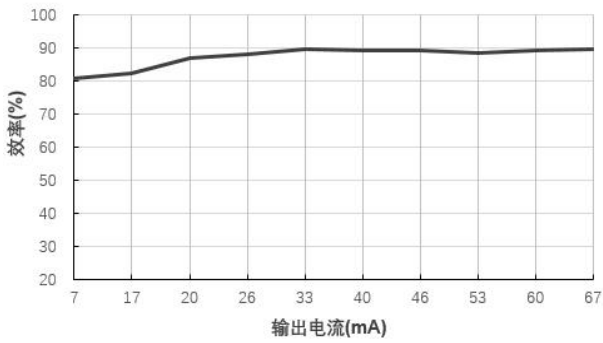
效率 VS 输出电流 (B1215S-1W@Vin=12V)
