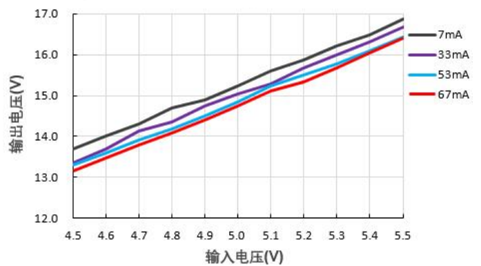
输出电压 VS 输入电压 (B0515S-1W)
