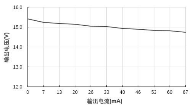
输出电压 VS 输出电流 (B0515S-1W@Vin=5V)
