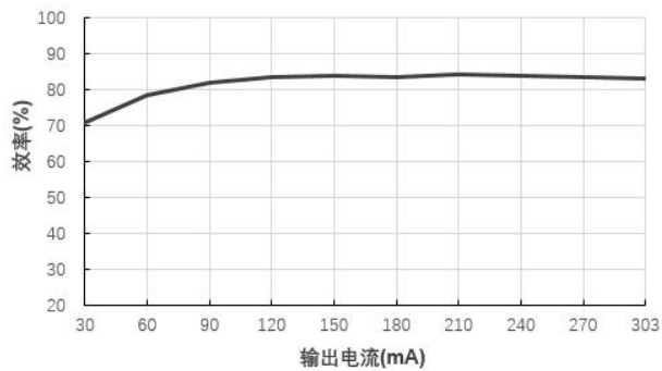
效率 VS 输出电流 (B0503S-1W@Vin=5V)
