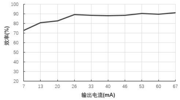
效率 VS 输出电流 (B2415S-1W@Vin=24V)
