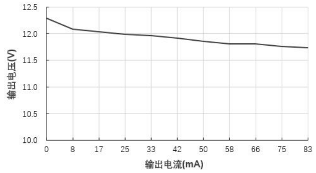
输出电压 VS 输出电流 (B1212S-1W@Vin=12V)
