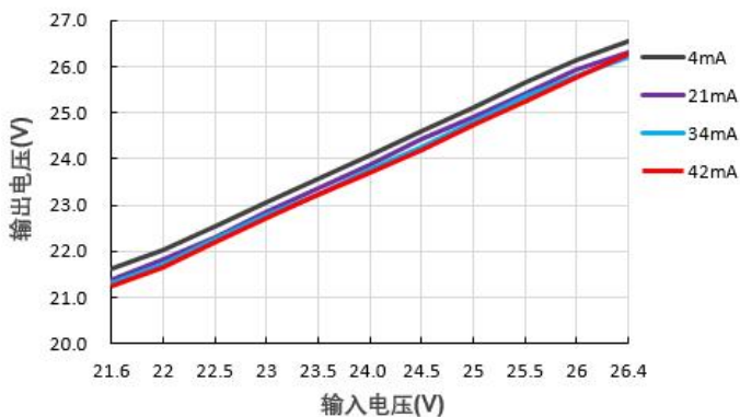
输出电压 VS 输入电压 (B2424S-1W)
