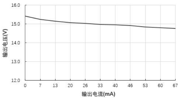
输出电压 VS 输出电流 (B1215S-1W@Vin=12V)
