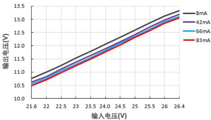
输出电压 VS 输入电压 (B2412S-1W)
