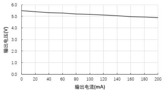
输出电压 VS 输出电流 (B0505S-1W@Vin=5V)
