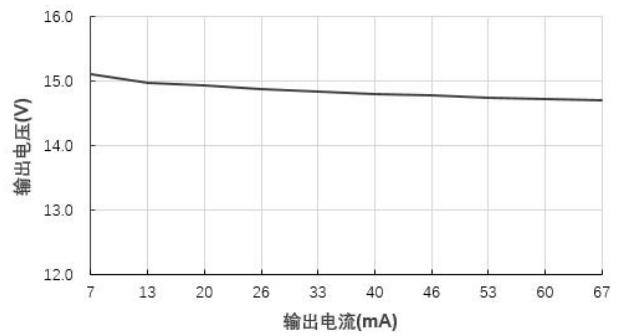
输出电压 VS 输出电流 (B2415S-1W@Vin=24V)
