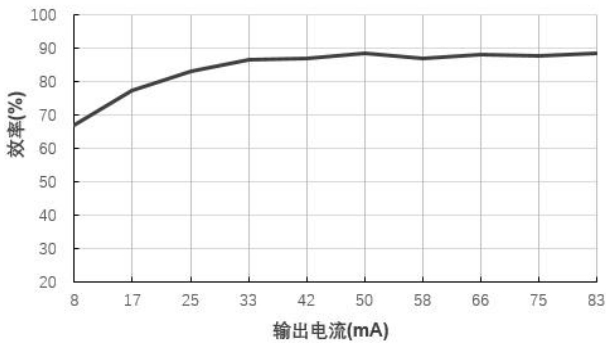
效率 VS 输出电流 (B2412S-1W@Vin=24V)
