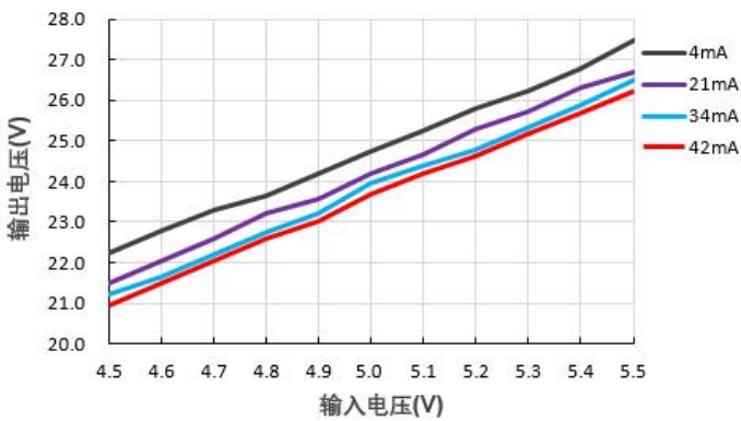
输出电压 VS 输入电压 (B0524S-1W)
