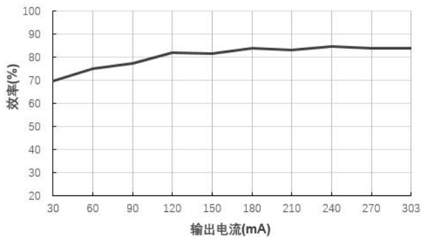
效率 VS 输出电流 (B2403S-1W@Vin=24V)
