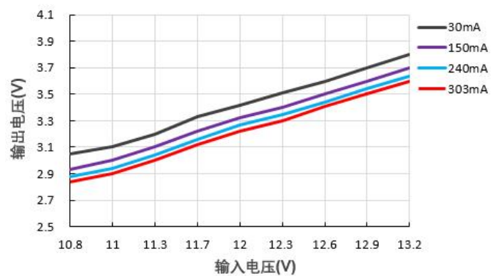
输出电压 VS 输入电压 (B1203S-1W)
