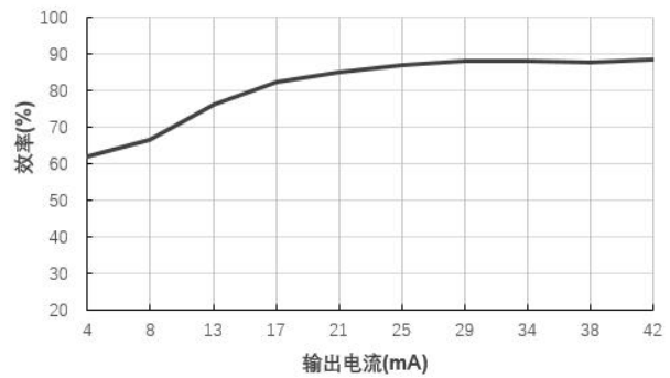
效率 VS 输出电流 (B1224S-1W@Vin=12V)
