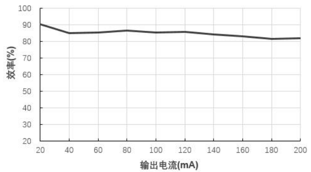
效率 VS 输出电流 (B0305S-1W@Vin=3.3V)
