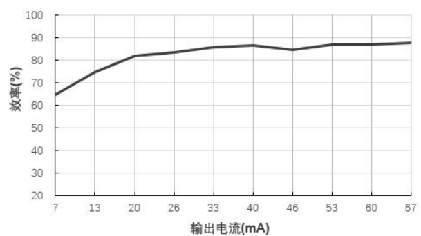
效率 VS 输出电流 (B0515S-1W@Vin=5V)
