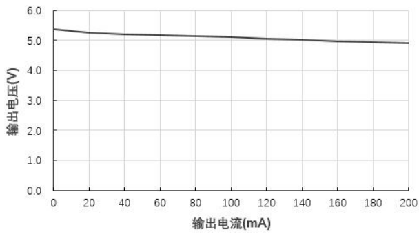
输出电压 VS 输出电流 (B1205S-1W@Vin=12V)
