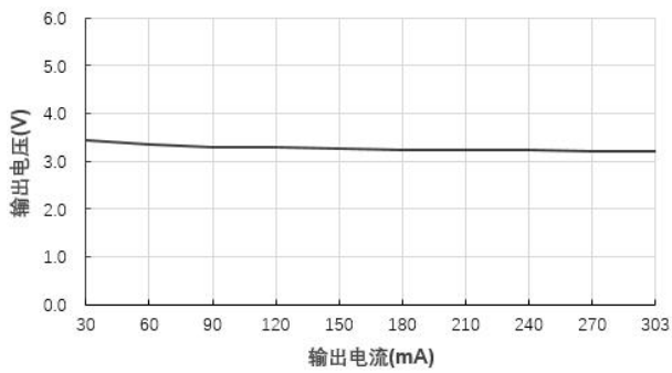
输出电压 VS 输出电流 (B2403S-1W@Vin=24V)
