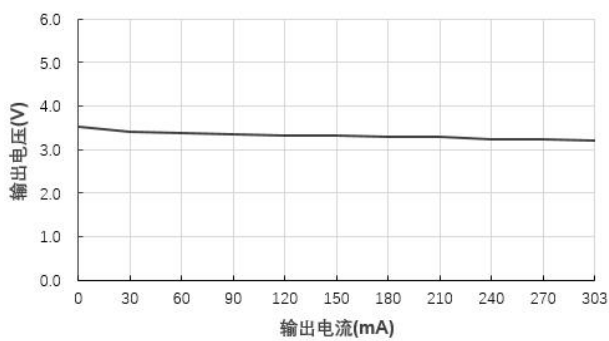
输出电压 VS 输出电流 (B0503S-1W@Vin=5V)
