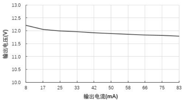
输出电压 VS 输出电流 (B2412S-1W@Vin=24V)
