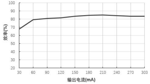
效率 VS 输出电流 (B1203S-1W@Vin=12V)
