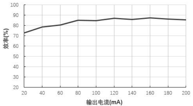
效率 VS 输出电流 (B2405S-1W@Vin=24V)
