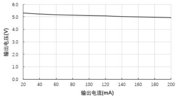
输出电压 VS 输出电流 (B2405S-1W@Vin=24V)
