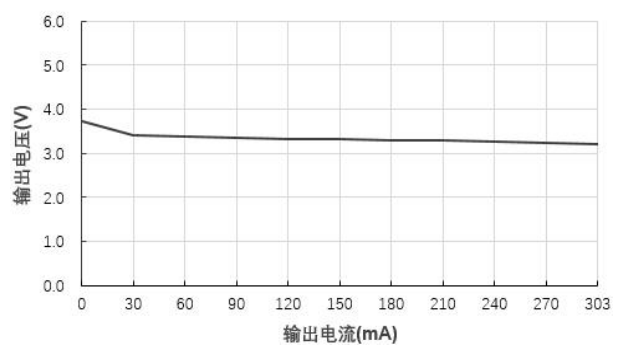
输出电压 VS 输出电流 (B1203S-1W@Vin=12V)
