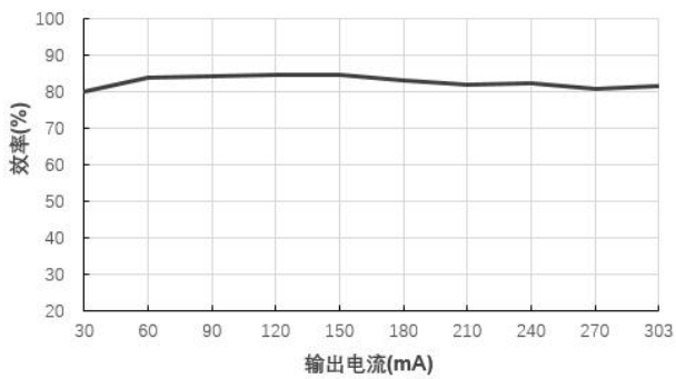
效率 VS 输出电流 (B0303S-1W@Vin=3.3V)
