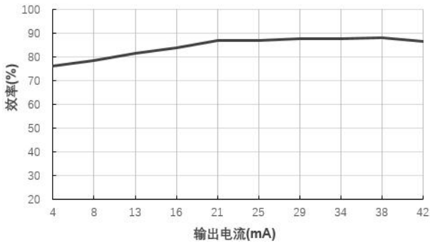
效率 VS 输出电流 (B0524S-1W@Vin=5V)
