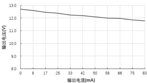
输出电压 VS 输出电流 (B0512S-1W@Vin=5V)
