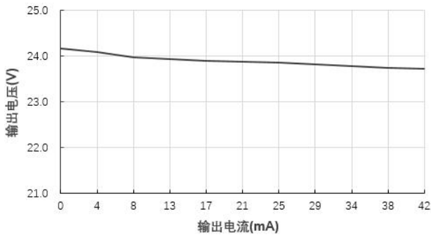
输出电压 VS 输出电流 (B2424S-1W@Vin=24V)
