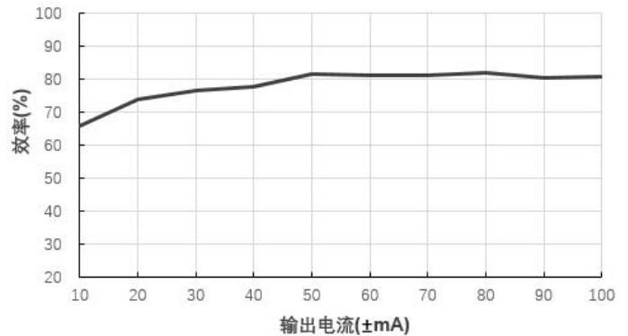
效率 VS 输出电流 A1205S-1W@ (Vin=12V)
