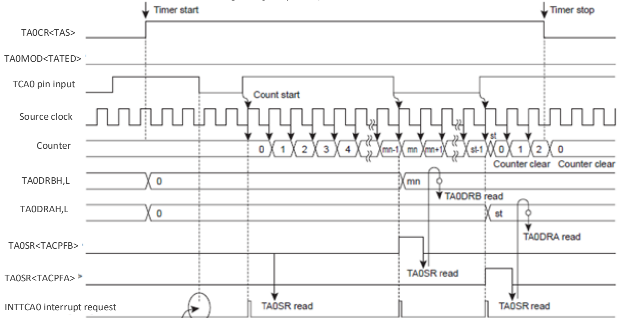
图 13- 10 脉宽测量模式时序图(TCA0 为范例)
