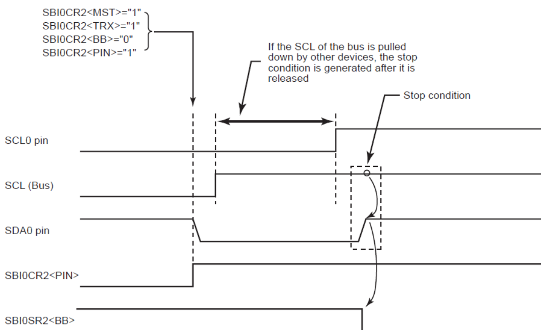
图 15-21 停止条件产生(以 SBI0 为范例)
