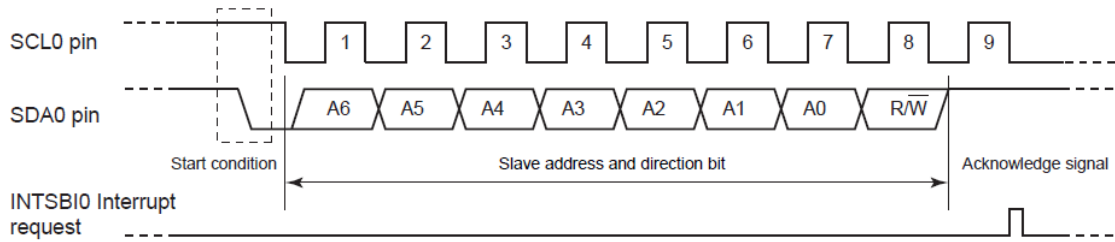
图 15-9 产生开始条件与从属地址(以 SBI0 为例)
