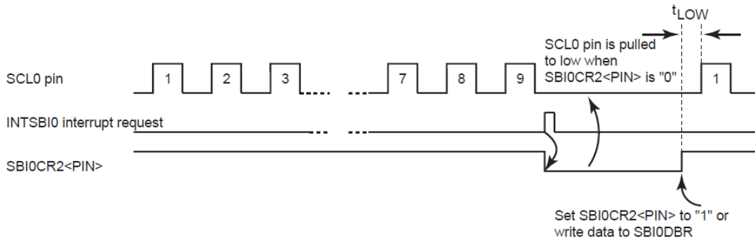
图 15- 11 SBIxCR2<PIN>与 SCLx 脚位(以 SBI0 为范例)
