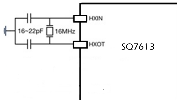
图 2-5 SQ7613 建议外部参考线路(使用外部参考时钟引脚)
