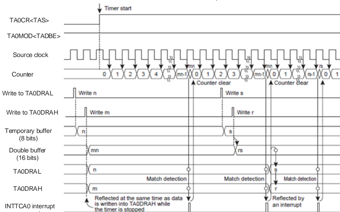
图 13- 10 定时器模式时序图(以 TCA0 为范例)
