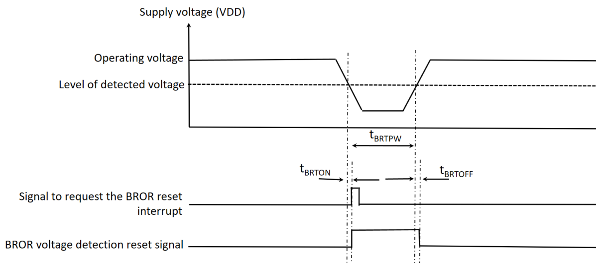
图 3-2 BROR 复位
