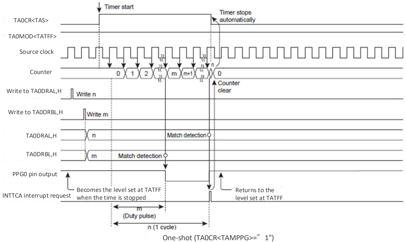
图 13- 17 PPG 模式时序图- 单次输出(TCA0 为范例)
