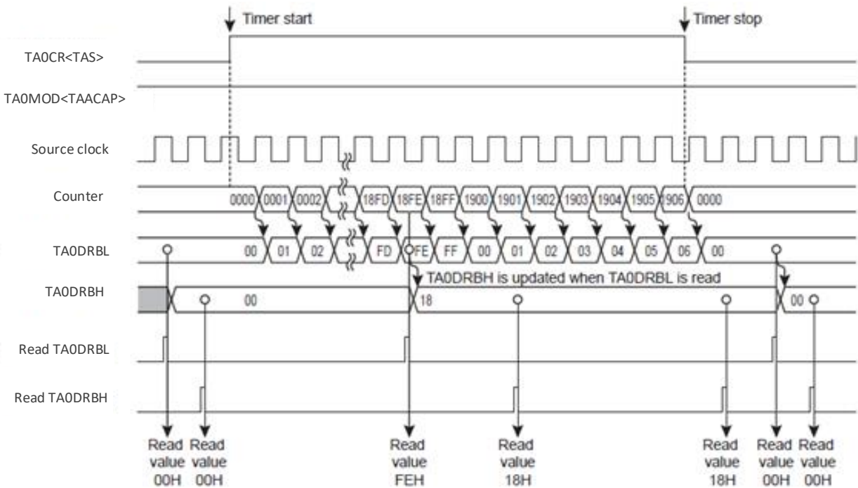
图 13- 11 TCA0 定时器模式范例时序图 (自动抓取)
