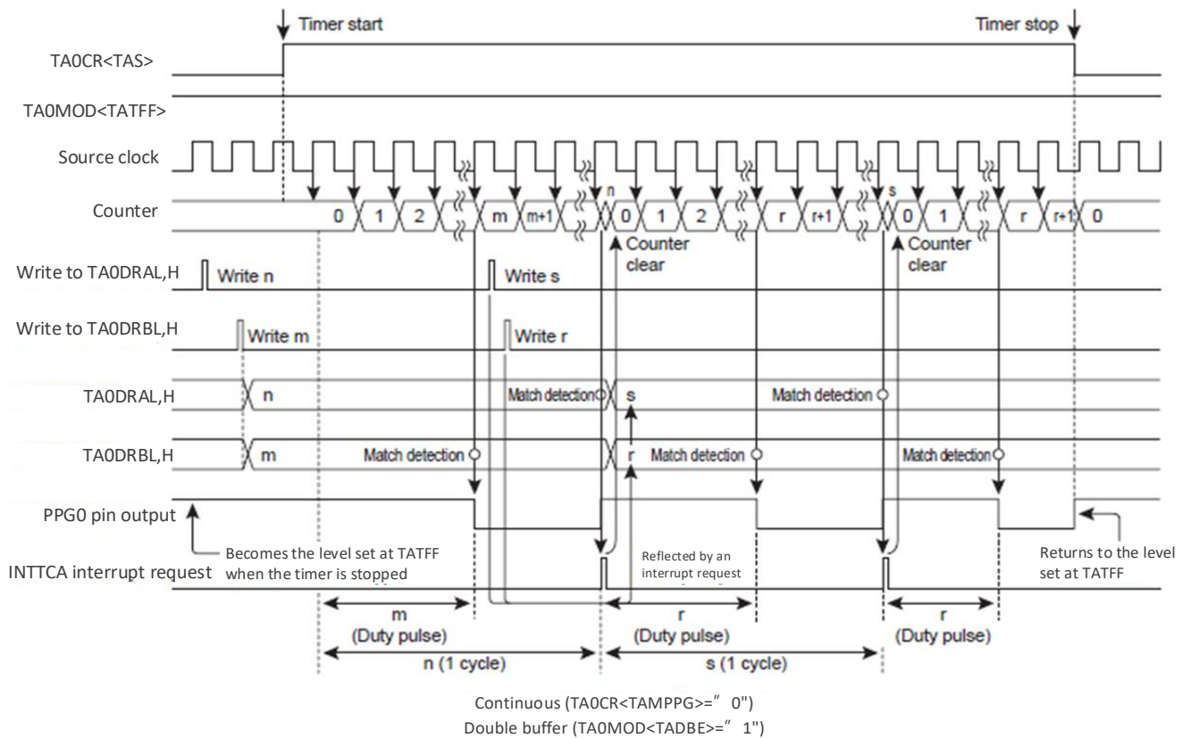
图 13- 18 PPG 模式时序图- 连续输出(TCA0 为范例)
