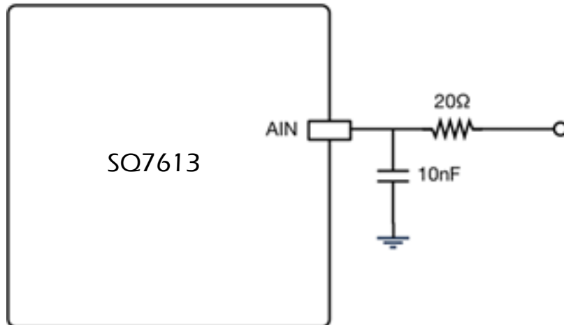
图 2-4 SQ7613 建议外部参考线路(进行 ADC 输入滤波)
