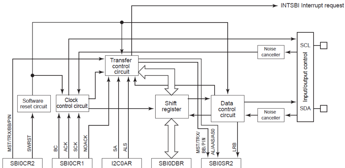
图 15-4 串行总线接口 0 (SBI0)方框图
