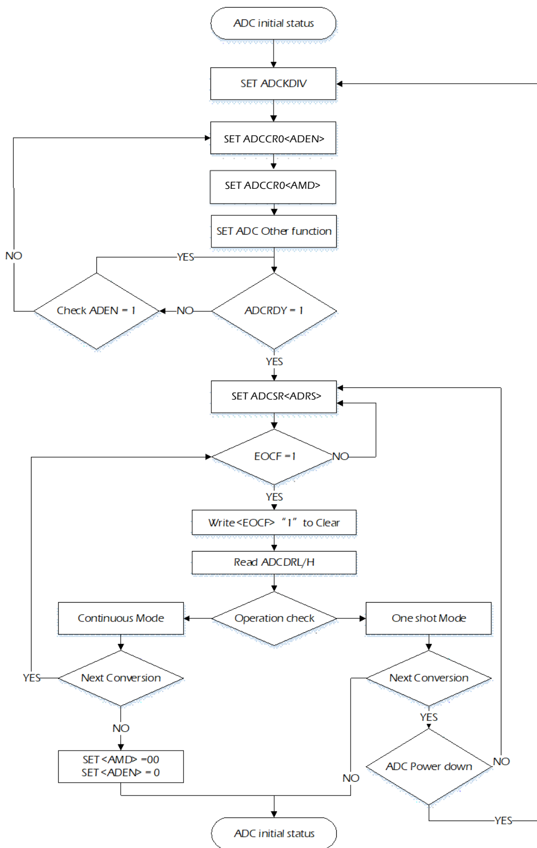
图 8-6 ADC 工作流程示意图
