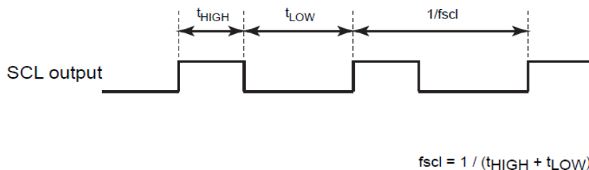
图 15-6 SCL 输出
