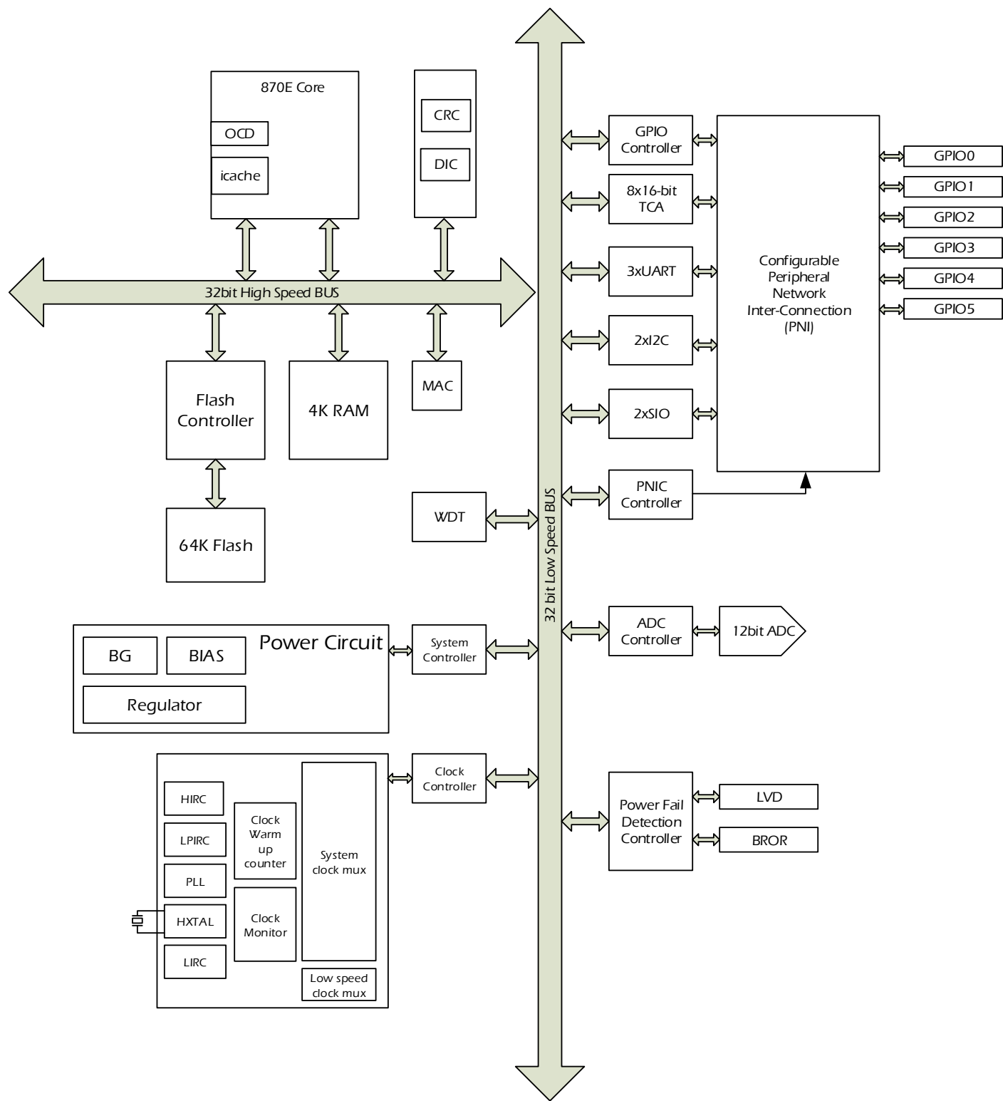
图 2-2 SQ7613 系统模块图
