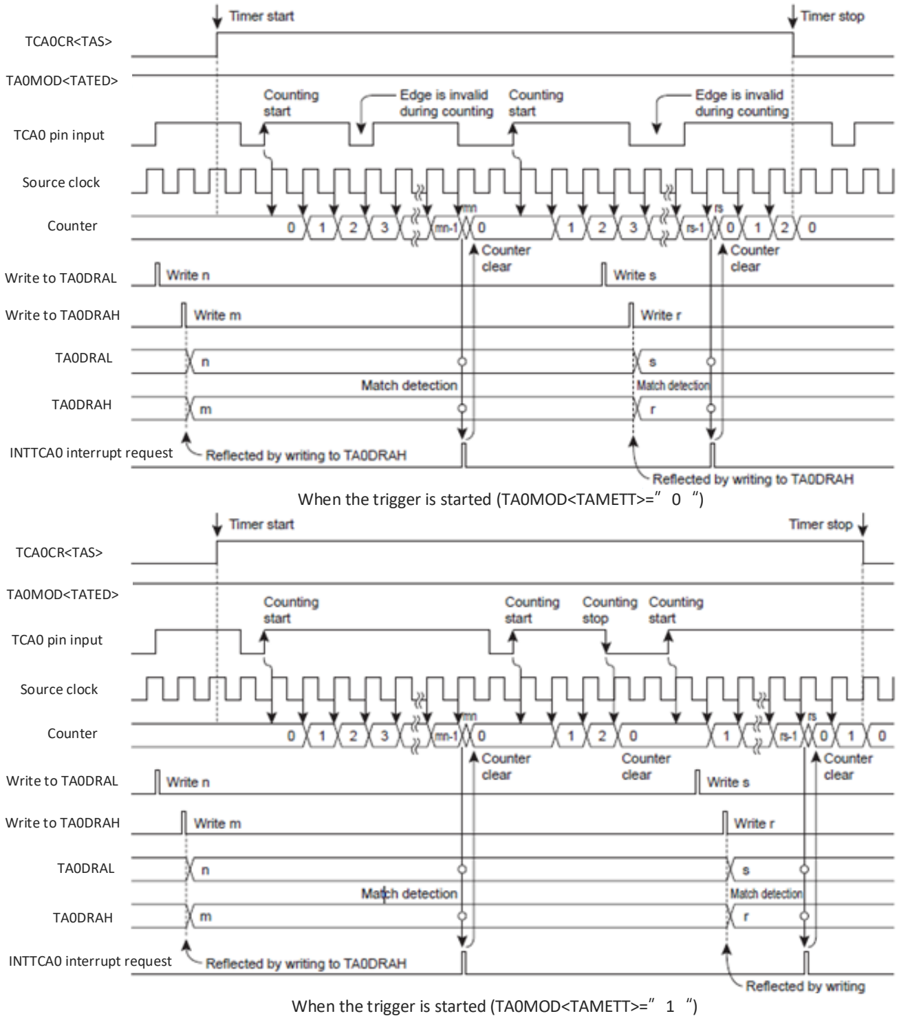
图 13-12 外部触发定时器模式时序图(TCA0 为范例)
