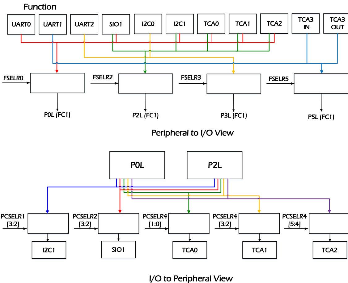
图 12-2 PNIC 架构图
