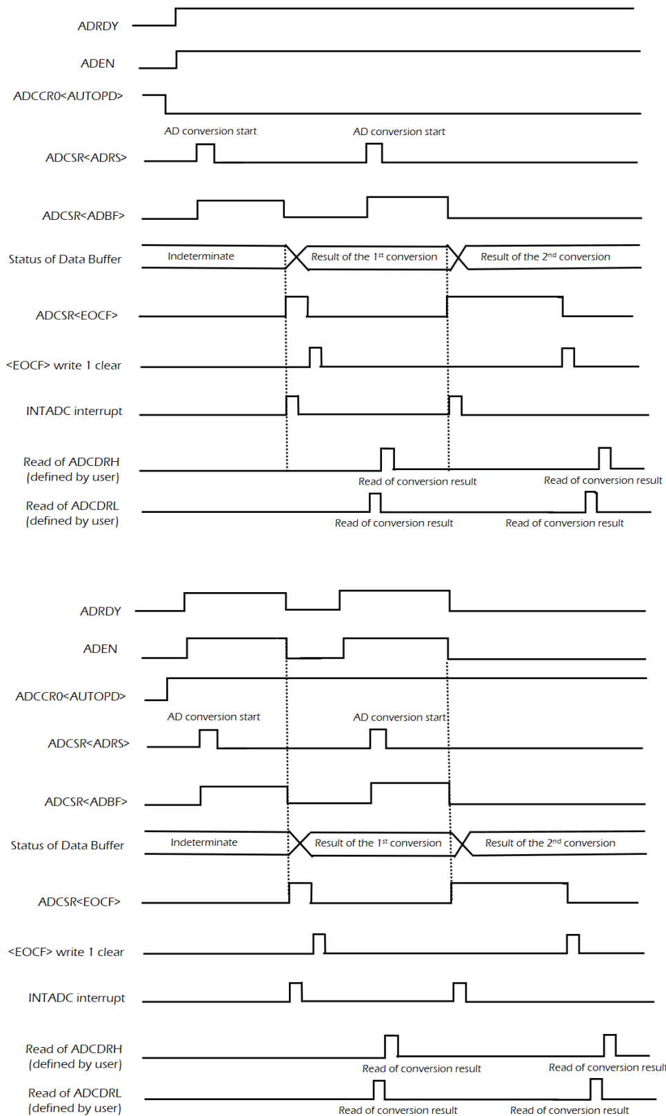
图 8-4 ADC 单次模式
