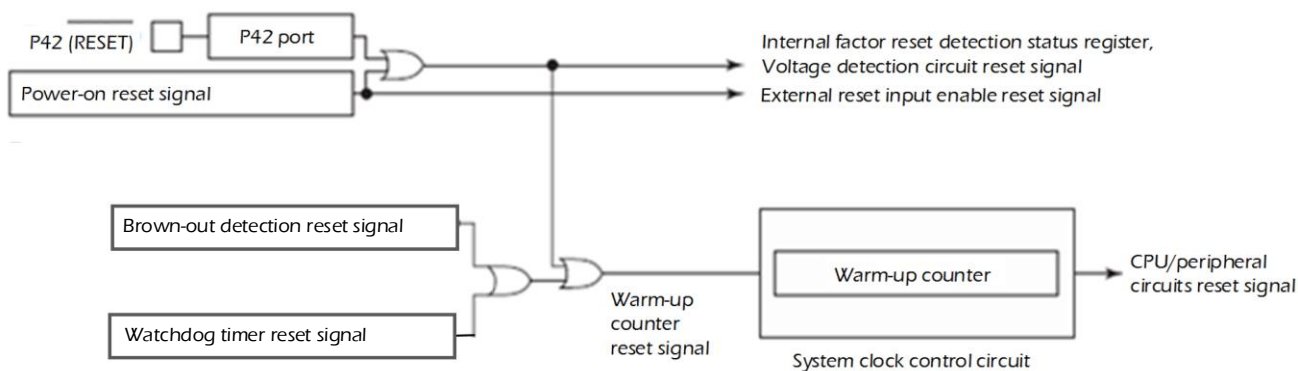
图 6-1 复位架构
