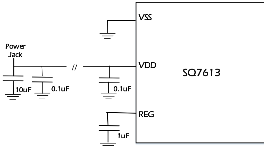
图 2-6 SQ7613 建议外部参考线路(电源去耦-POWER DECOUPLING)
