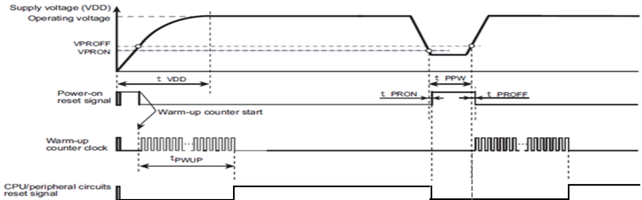
图 3-1 上电复位时序图
