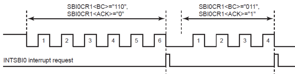
图 15- 5 数据传输时的时钟脉冲与 SBIxCR1<BC>, SBIxCR1<ACK>(图以 SBI0 作为范例)
