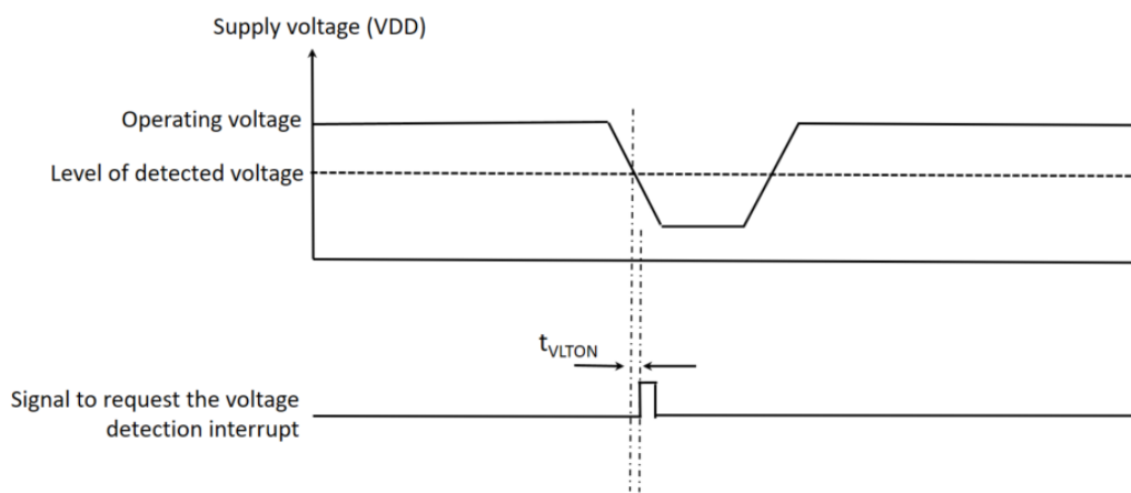
图 3-3 LVD 中断
