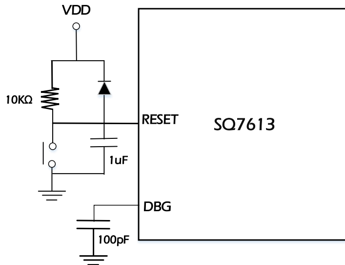
图 2-7 SQ7613 建议外部参考线路(复位引脚与仿真引脚)
