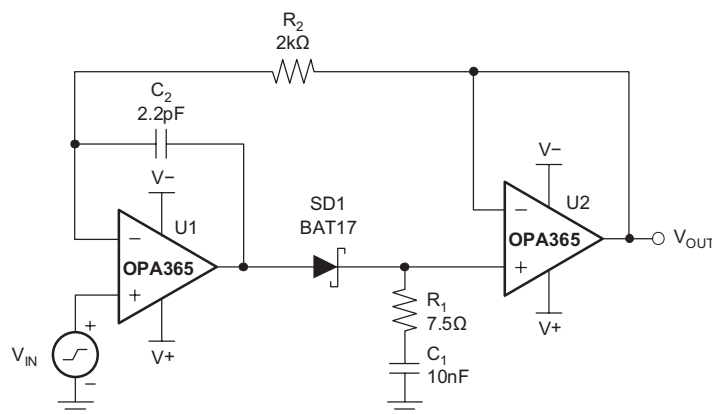
快速趋稳峰值检测器
