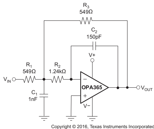
图 24. 二阶巴特沃斯 500kHz 低通滤波器
