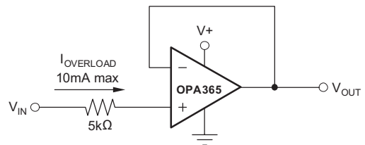
图 21. 输入电流保护
