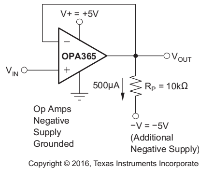
图 23. 摆动到接地
