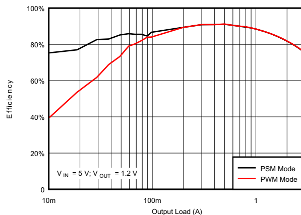
效率与输出负载之间的关系
