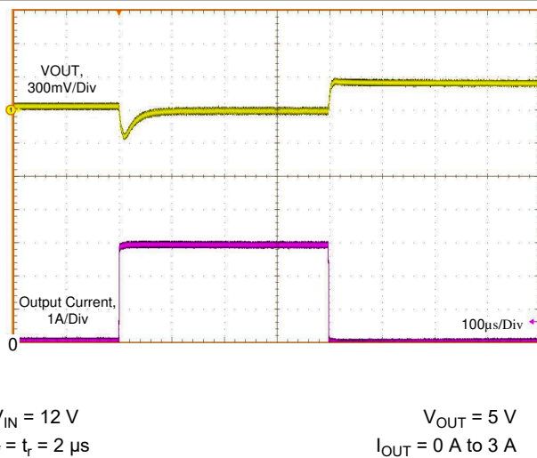
图 9-23. Load Transient
