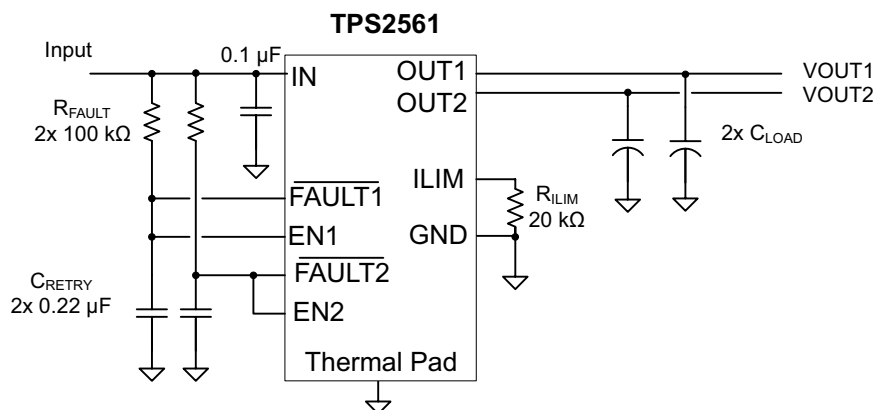
图 10-1. Auto-Retry Functionality
