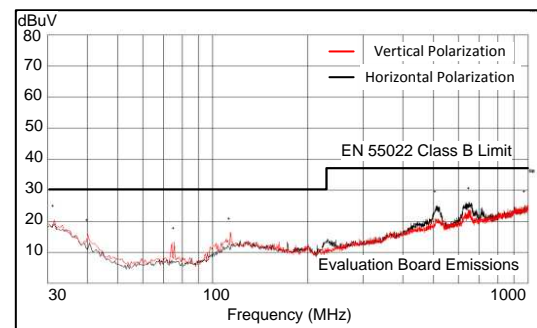
辐射发射图
