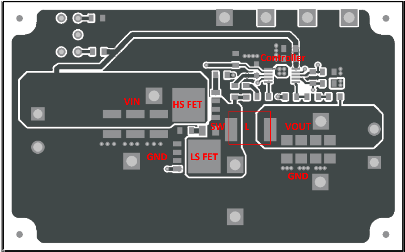
图 21. TPS53015 Layout
