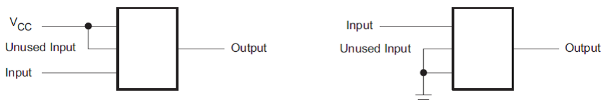
图 10-1. Layout Example
