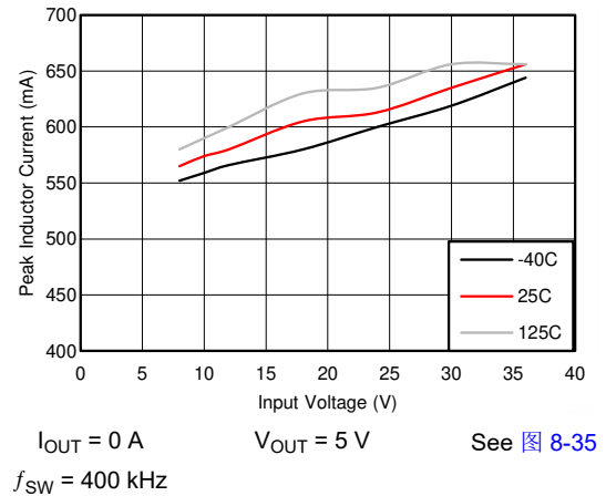
图 6-6. I PEAK-MIN
